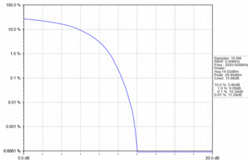
n41_15kHz_SISO_NTNV_30MHz_DFT-s-OFDM_PI/2_BPSK_2593.005MHz_Outer_Full
