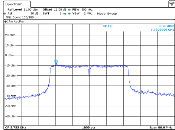
802.11ac40_5755MHz
