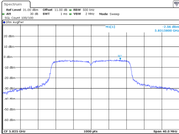
802.11ac20_5825MHz
