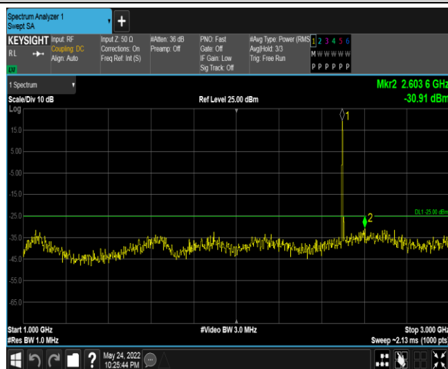
Band41-10MHz-QPSK-39700-1RB#0-Range2:1000~3000MHz
