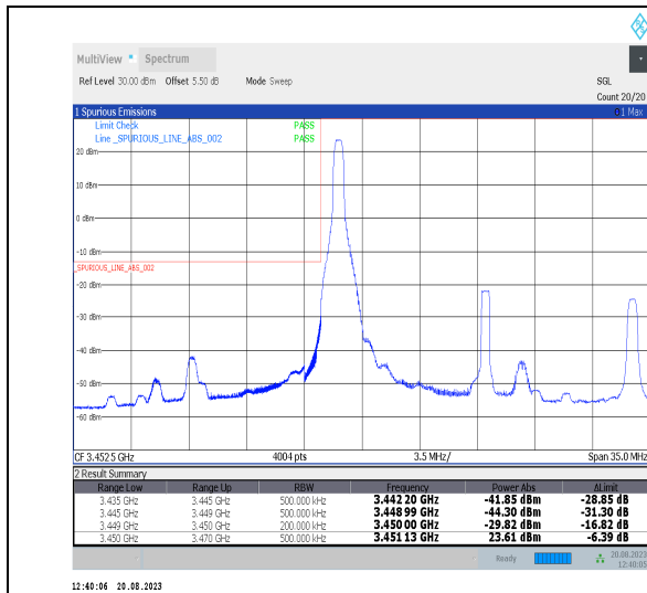
Band42_20MHz_QPSK_42190_1RB#0
