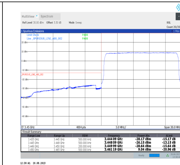
Band42_15MHz_QPSK_42165_75RB#0
