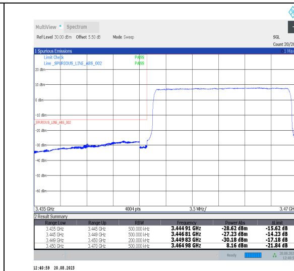
Band42_20MHz_QPSK_42190_100RB#0
