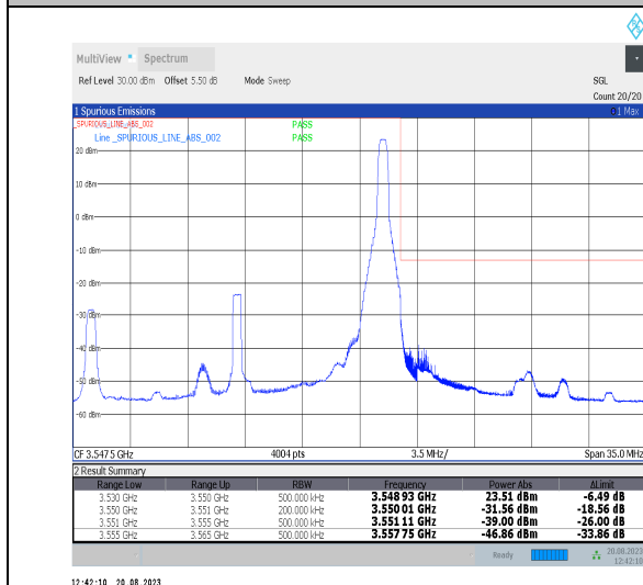
Band42_20MHz_QPSK_42990_1RB#99
