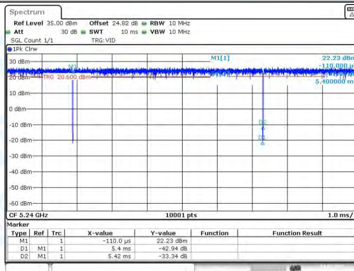
11A_Ant3_5240
