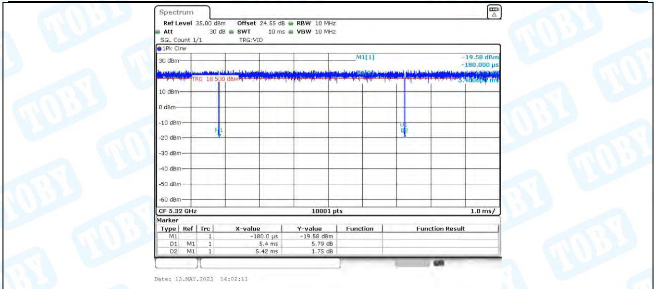
11A_Ant2_5320
