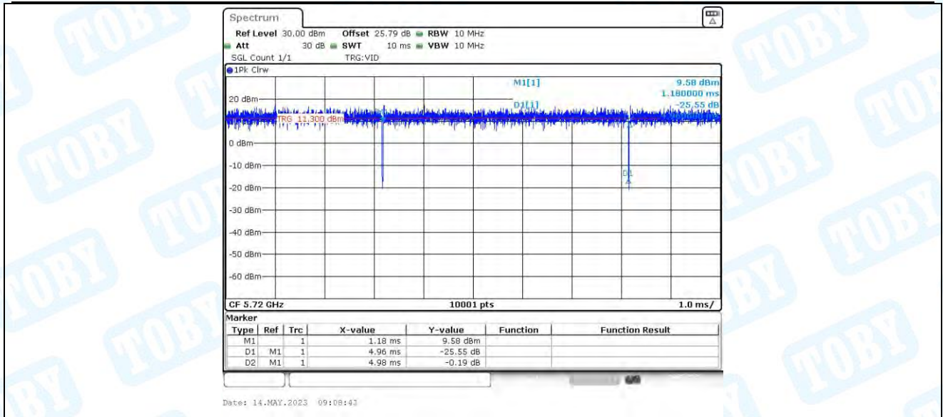
11N20MIMO_Ant3_5720
