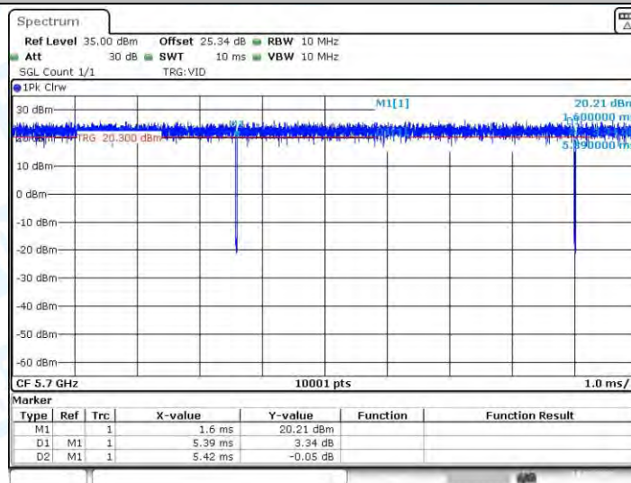
11A_Ant3_5700
