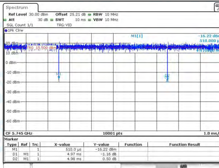
11N20MIMO_Ant3_5745
