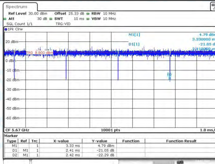
11N40MIMO_Ant3_5670
