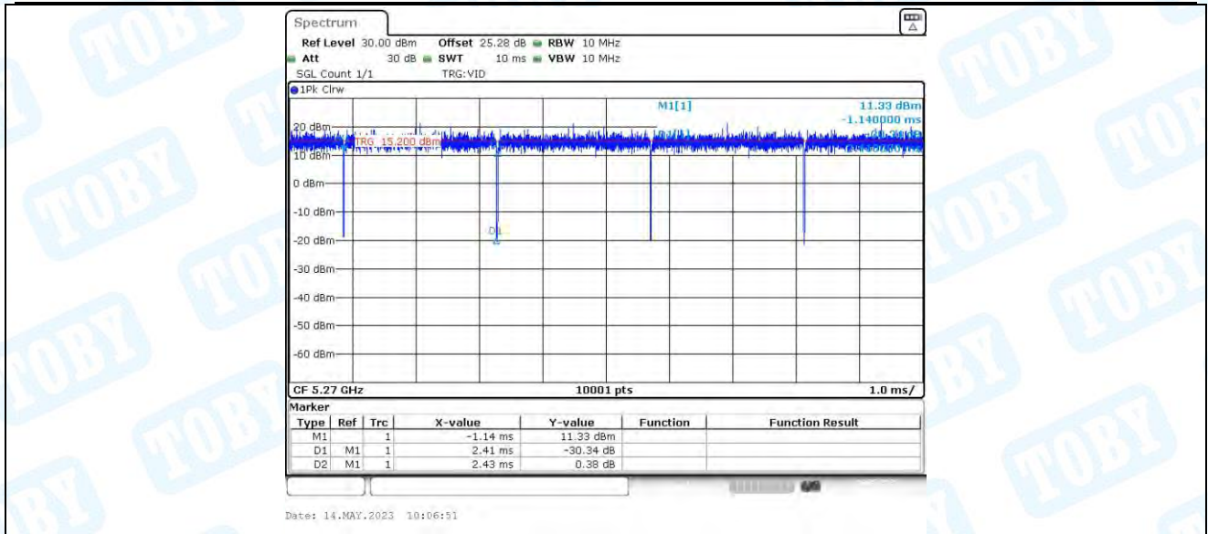
11N40MIMO_Ant3_5270
