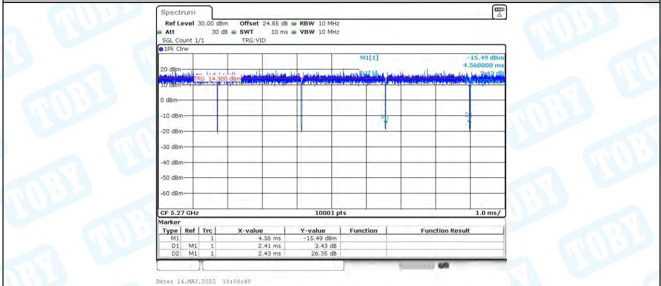
11N40MIMO_Ant4_5270
