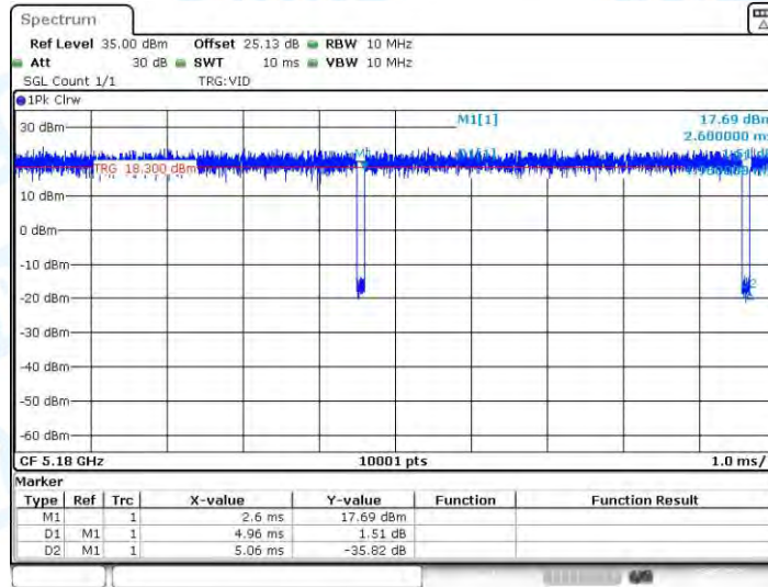
11N20MIMO_Ant3_5180
