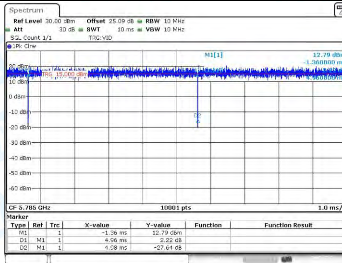
11N20MIMO_Ant4_5785
