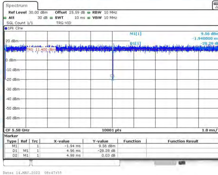
11N20MIMO_Ant3_5580
