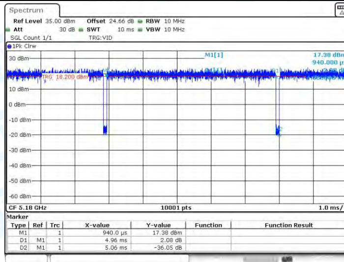
11N20MIMO_Ant3_5180
