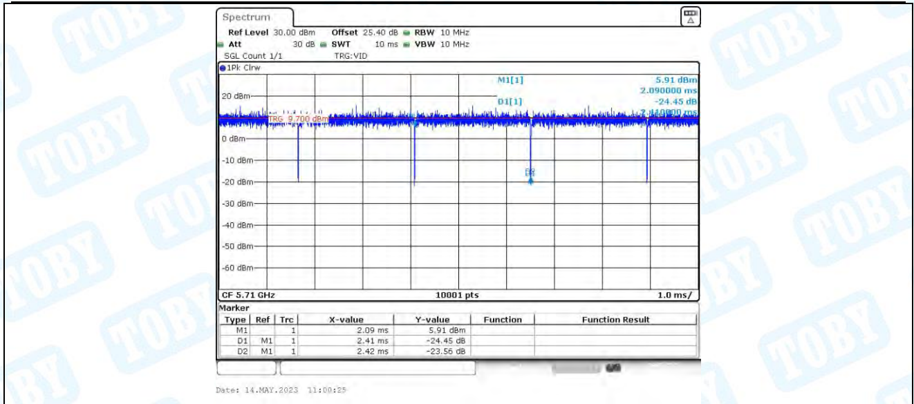
11N40MIMO_Ant4_5710
