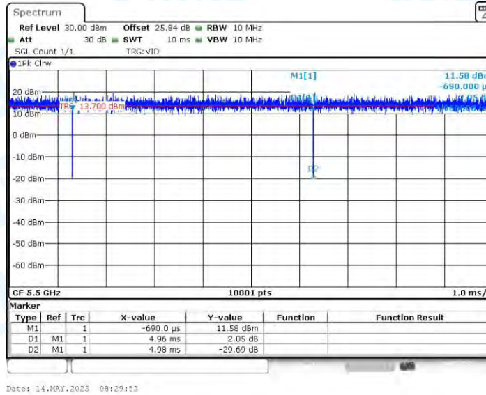
11N20MIMO_Ant3_5500
