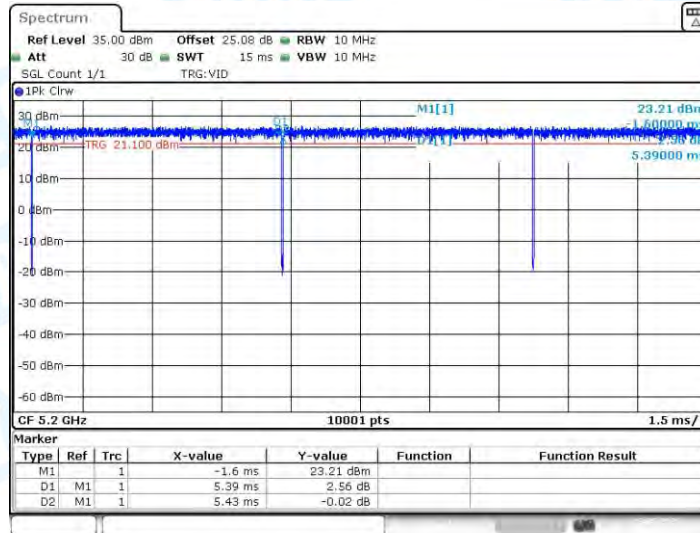
11A_Ant3_5200
