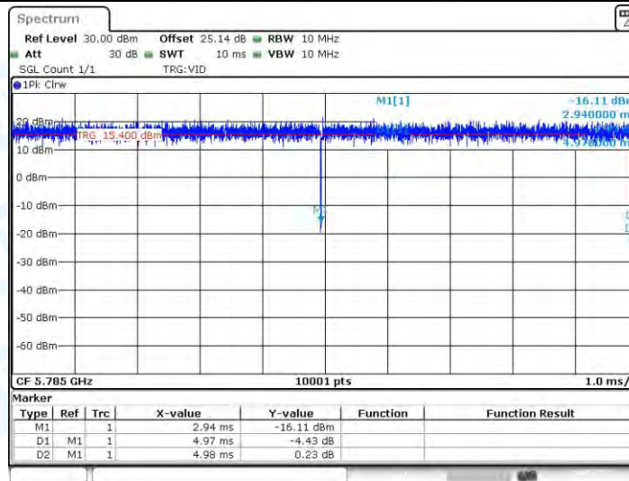
11N20MIMO_Ant4_5785
