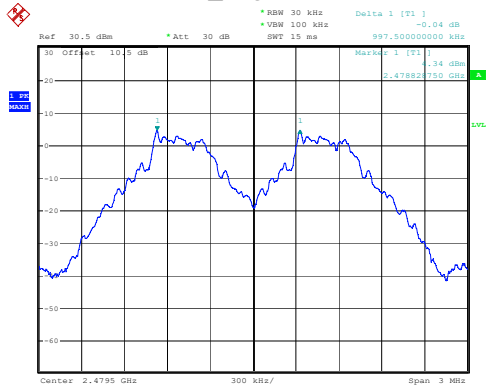
DH1_High 0.998MHz
