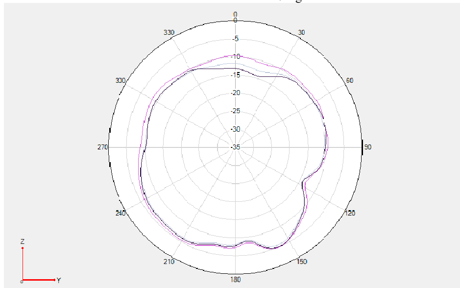
LTE B1&N1 \Phi=90^\circ
