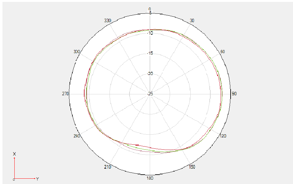
GSM850/WCDMA B5/LTE B5/N5 \Theta=90^\circ
