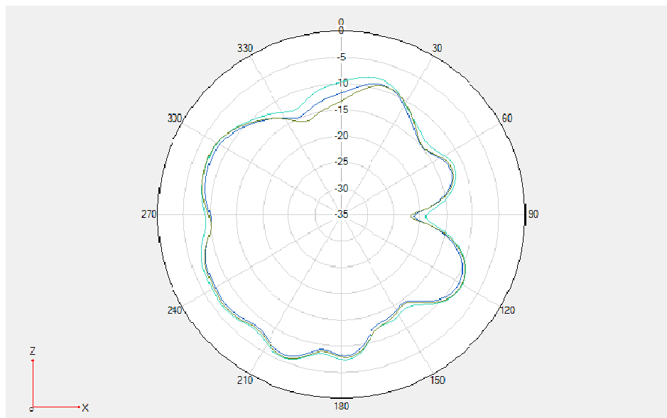
LTE B1&N1 \Phi=0^\circ
