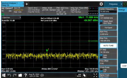
Band25-20MHz-QPSK-26365-1RB#0-0.009~0.15-PASS
