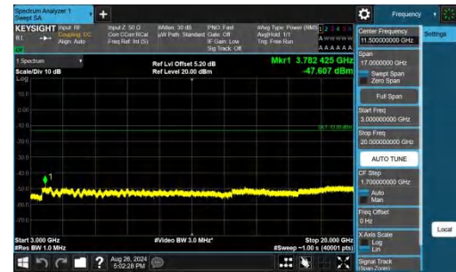
Band25-20MHz-QPSK-26365-1RB#99-3000~20000-PASS
