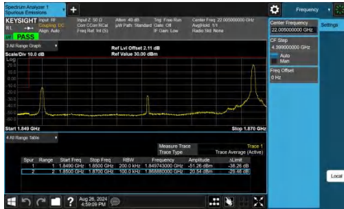
Band25-20MHz-QPSK-26140-1RB#99-PASS
