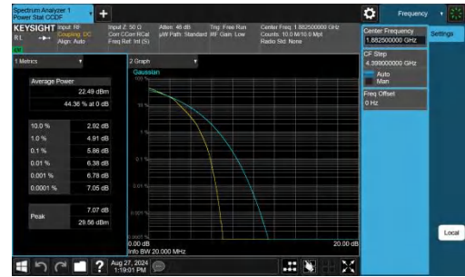
Band25-20MHz-16QAM-26365-27RB#0-PASS
