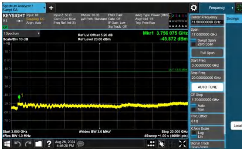
Band25-10MHz-QPSK-26365-1RB#0-3000~20000-PASS
