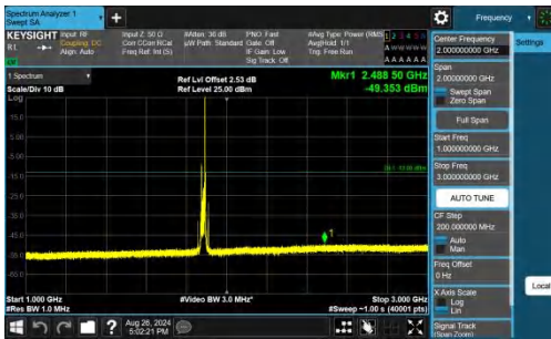
Band25-20MHz-QPSK-26365-1RB#99-1000~3000-PASS
