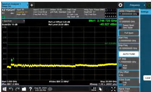
Band25-20MHz-QPSK-26365-1RB#0-3000~20000-PASS
