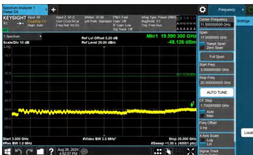
Band25-15MHz-QPSK-26115-1RB#0-3000~20000-PASS
