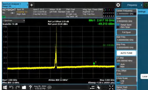
Band25-20MHz-QPSK-26590-1RB#99-1000~3000-PASS
