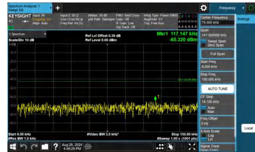
Band25-10MHz-QPSK-26365-1RB#49-0.009~0.15-PASS
