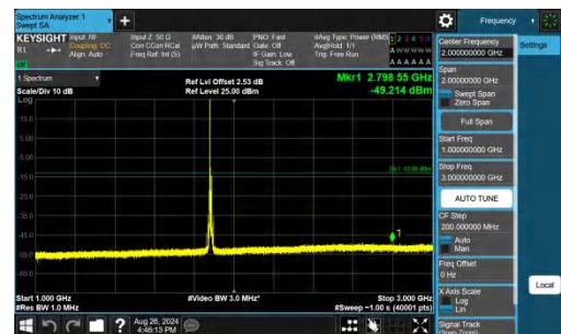
Band25-10MHz-QPSK-26365-1RB#0-1000~3000-PASS
