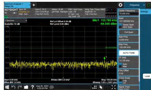
Band25-20MHz-QPSK-26365-1RB#99-0.009~0.15-PASS
