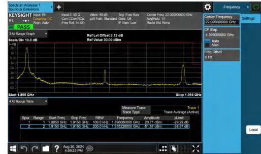
Band25-20MHz-QPSK-26590-1RB#0-PASS
