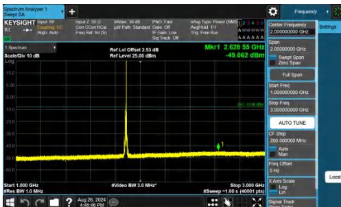
Band25-10MHz-QPSK-26365-1RB#49-1000~3000-PASS
