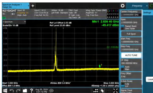
Band25-20MHz-QPSK-26140-1RB#99-1000~3000-PASS
