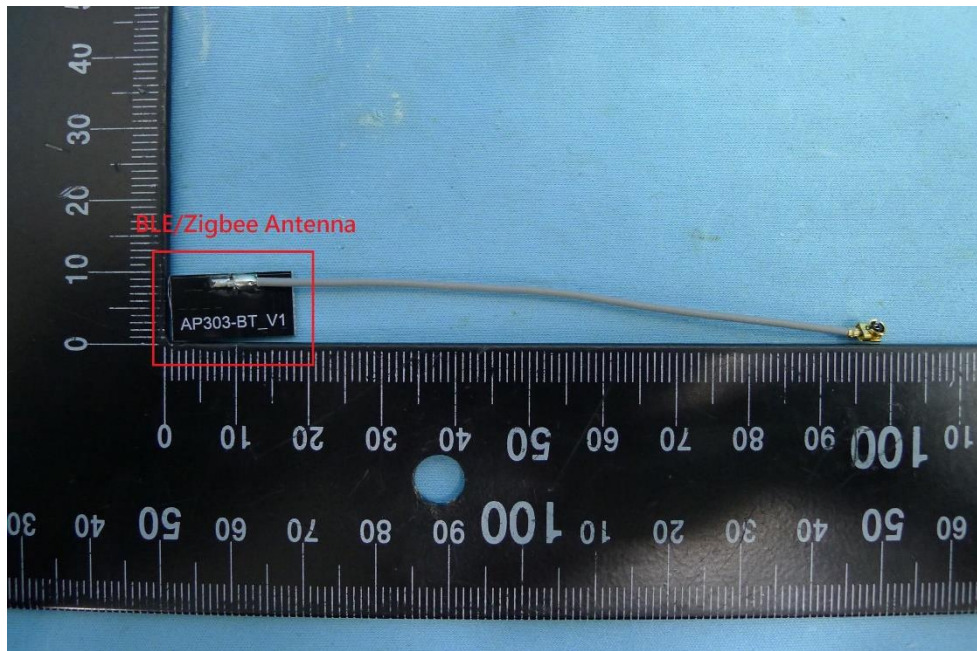
(14) EUT Photo
