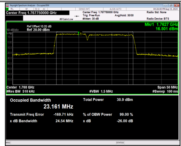
66-66-10MHz-15MHz-QPSK-QPSK-132477-132597-50RB #0-75RB#0-PASS
