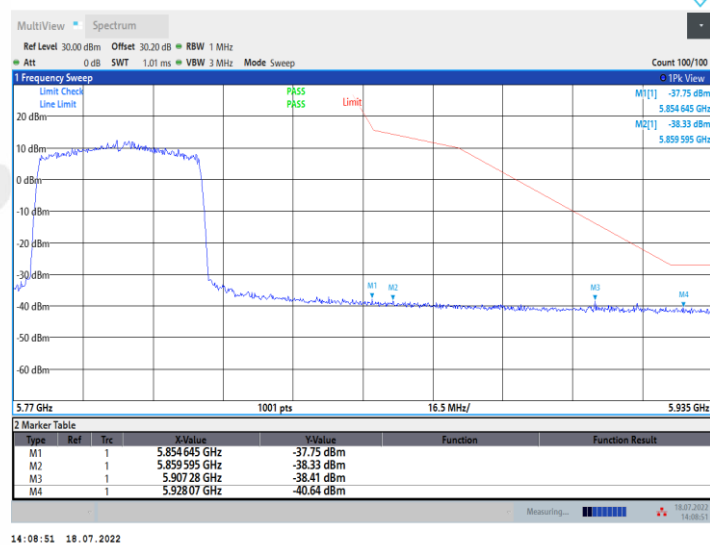
11AX80MIMO_Low_5775
