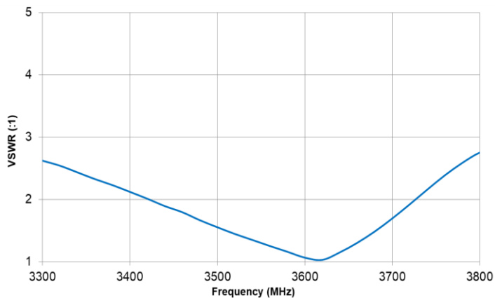
VSWR
