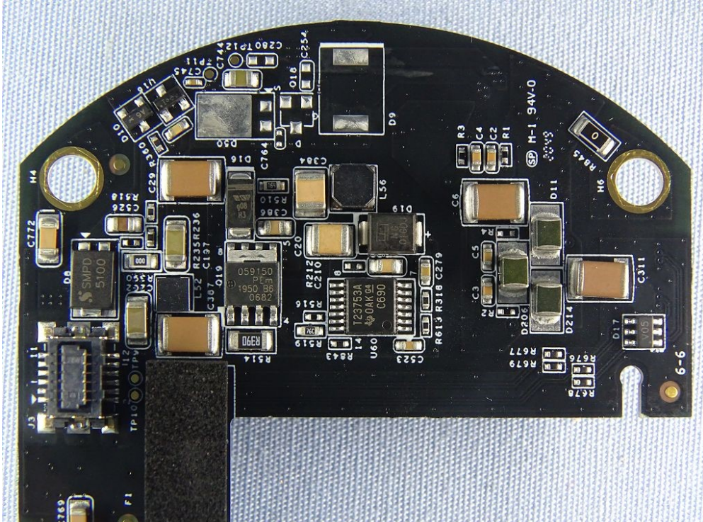
(8) EUT Photo
