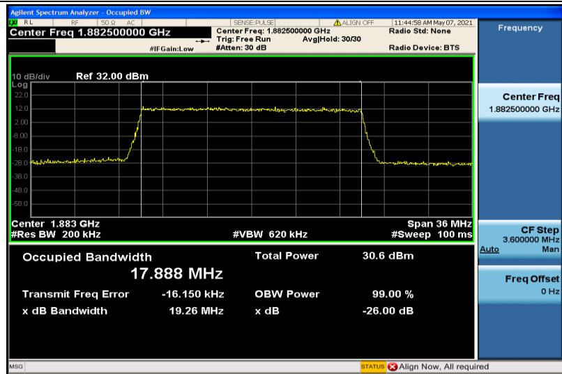
Band25-20MHz-QPSK-26365-100RB#0-17.888
