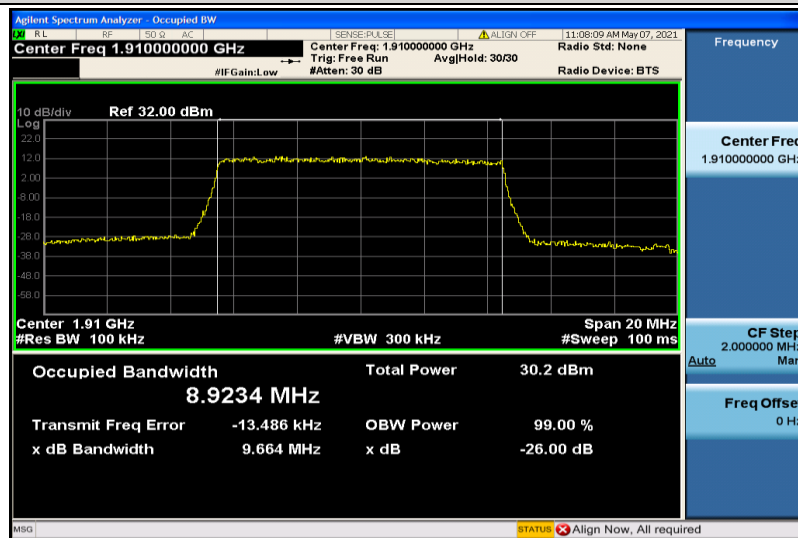
Band25-10MHz-QPSK-26640-50RB#0-8.9234
