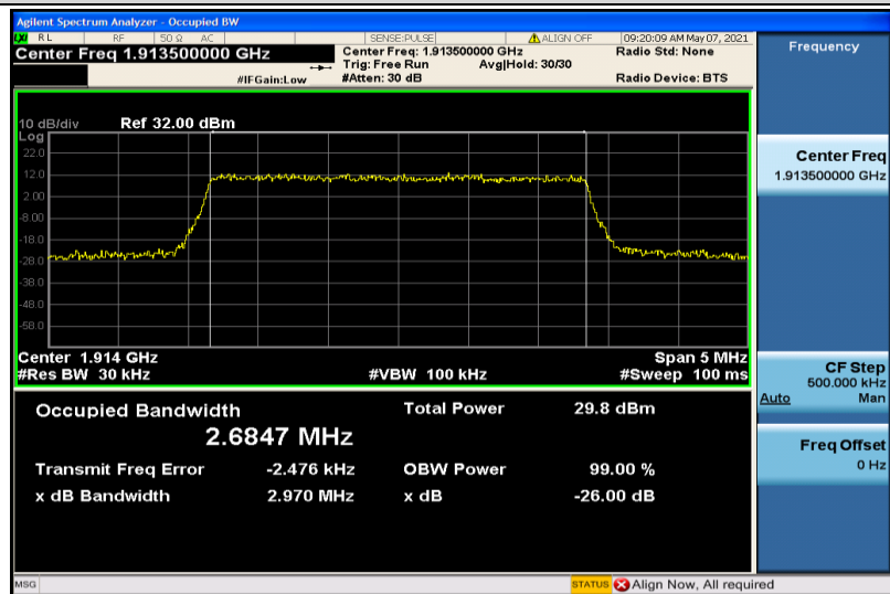
Band25-3MHz-QPSK-26675-15RB#0-2.6847
