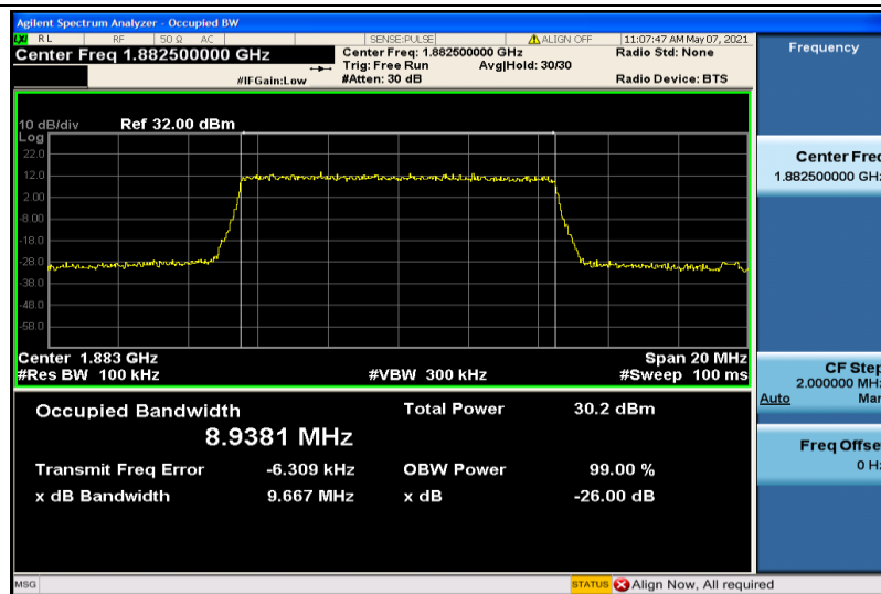
Band25-10MHz-QPSK-26365-50RB#0-8.9381
