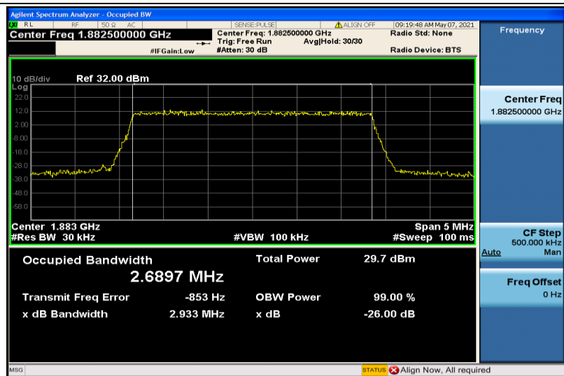
Band25-3MHz-QPSK-26365-15RB#0-2.6897
