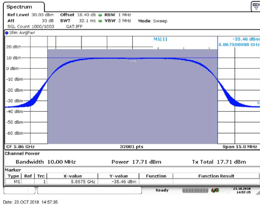
Antenna 1, Ch. 172 (SISO)
