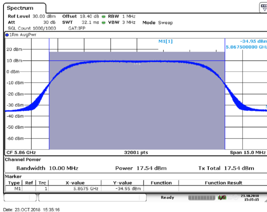
Antenna 2, Ch. 172 (SISO)
