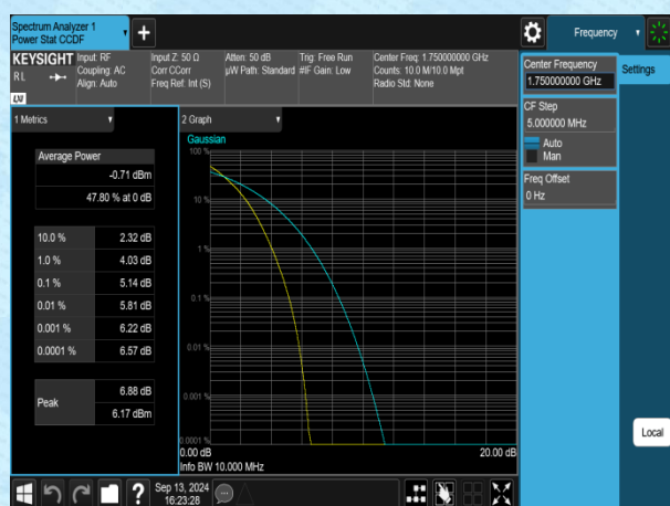
Band4-10MHz-QPSK-20350-1RB#0-PASS
