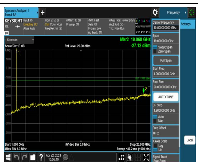
Band4-1.4MHz-QPSK-20175-1RB#0-Range2:1000~20
