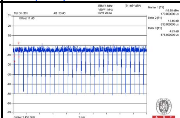
802.11n (40MHz)
