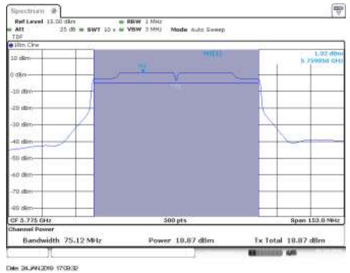
SISO B, CH155, 802.11ac80, VHT0
