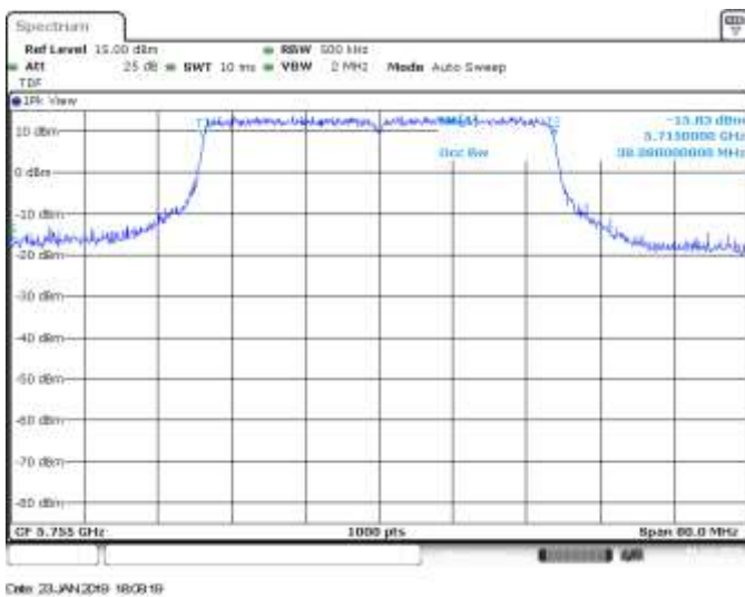
SISO A, CH151, 802.11ax40, HE0, 99%
