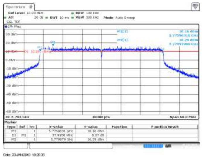
MIMO A, CH159, 802.11ax40, HE0, 6dB
