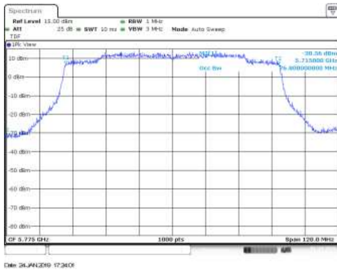
SISO B, CH155, 802.11ax80, HE0, 99%
