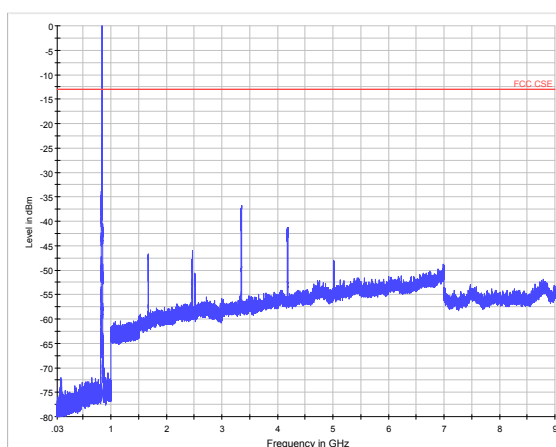
WCDMA Band V CH-High 30MHz ~ 9GHz
