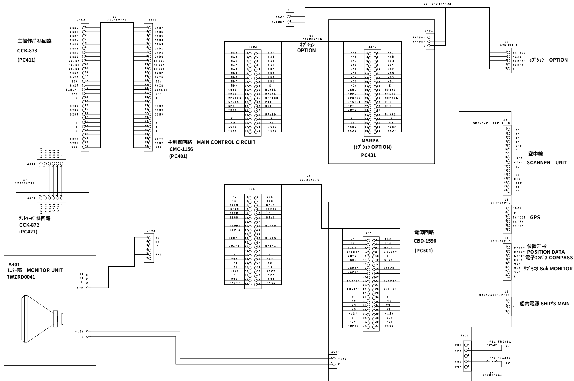
【図 1 1 1 NCD-4170 指示機機内接続図】 【Fig.111 INTERNAL CONNECTIONS OF DISPLAY UNIT NCD-4170】
