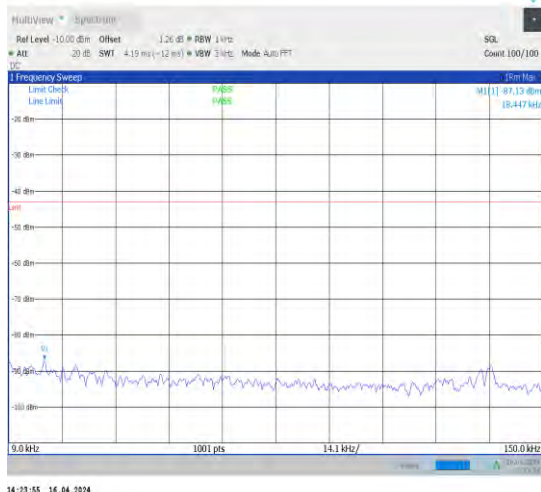
1-N78-3700-3800-N78-3700-380030-100-L-1-DFT-P I2BPSK-Inner_1RB_Left-1@1-0.009-0.15-Ant1-0.01 --87.13--43-PASS
