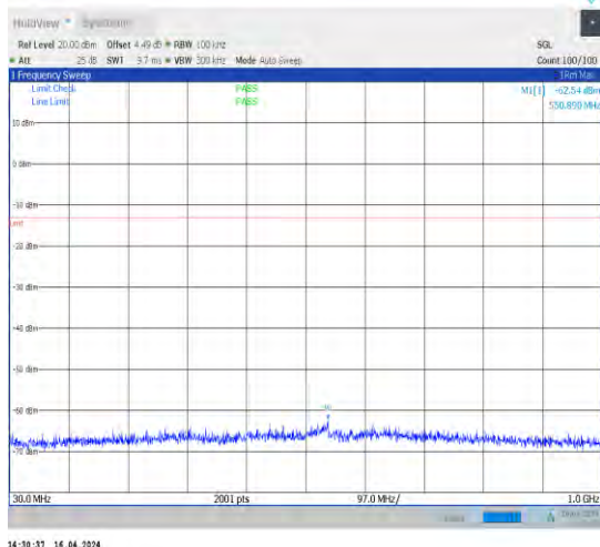
1-N78-3700-3800-N78-3700-380030-100-L-1-DFT-P I2BPSK-Inner_1RB_Left-1@1-30-1000-Ant1-529.55 --62.54--13-PASS
