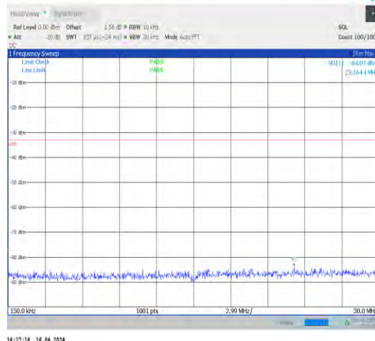
1-N78-3700-3800-N78-3700-380030-100-L-1-DFT-PI 2BPSK-Inner_1RB_Left-1@1-0.15-30-Ant1-28.60--8 4.07--33-PASS
