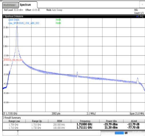
Band4-20MHz-QPSK-20050-1RB#99-PASS
