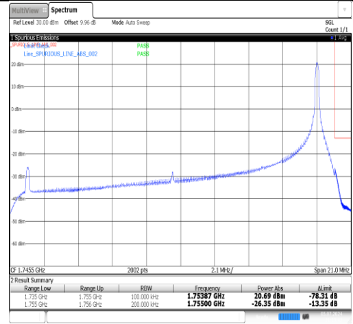
Band4-20MHz-QPSK-20300-1RB#99-PASS
