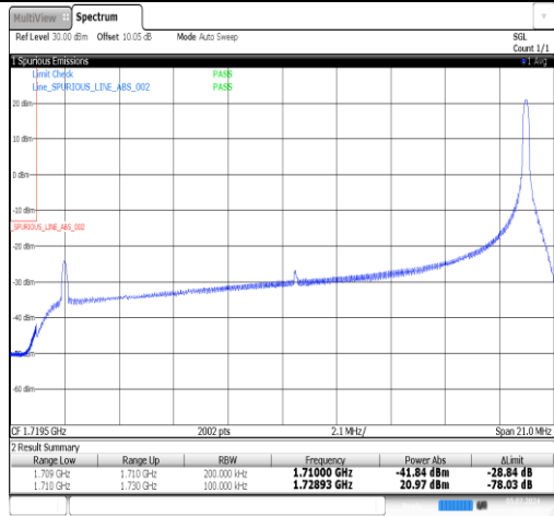
Band4-20MHz-QPSK-20050-1RB#99-PASS
