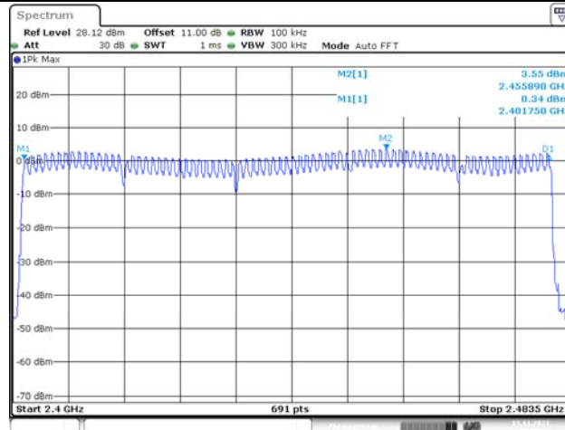
3DH1_Ant1_Hop
