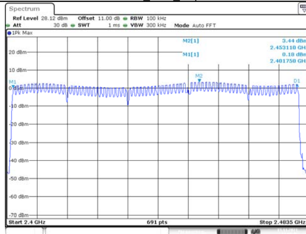
2DH1_Ant1_Hop
