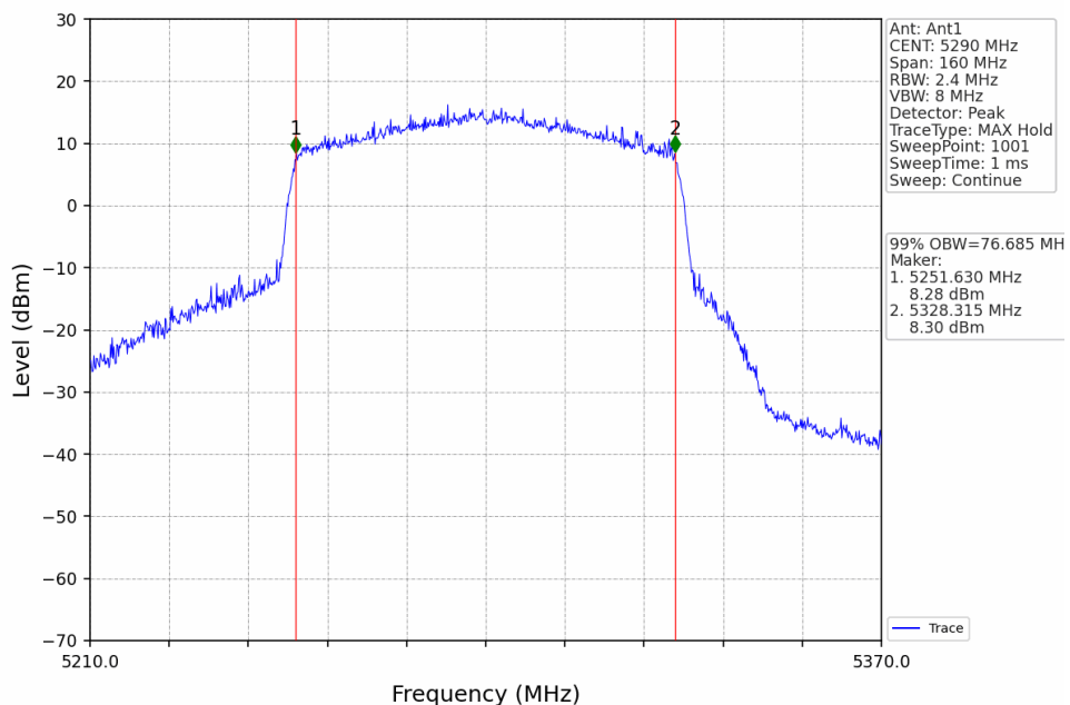
802.11ax(HEW80)_MCH_5290MHz_RU996_Left_Ant1_NTNV
