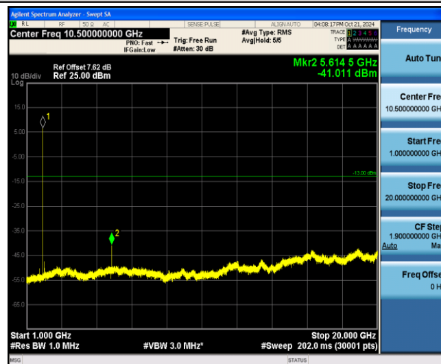
Band2-20MHz-16QAM-18900-1-0-Low-1000-20000--41.01-PASS
