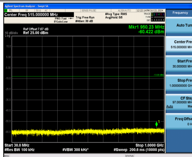
Band4-1.4MHz-QPSK-19957-1-0-Low-30-1000--60.42-PASS
