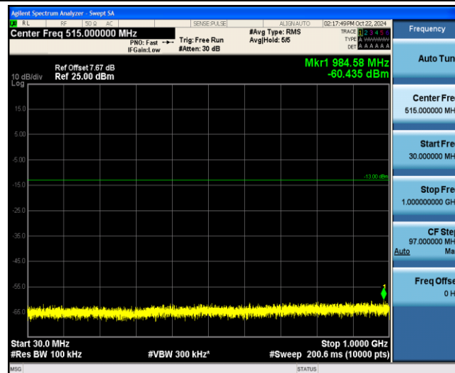
Band4-10MHz-QPSK-20000-1-0-Low-30-1000--60.44-PASS
