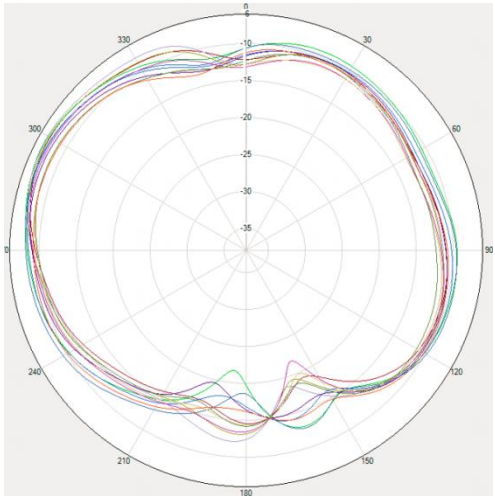
LTE B40 Theta=90deg
