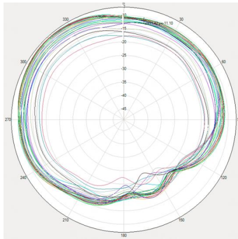
LTE B1/B66 Theta=90deg
