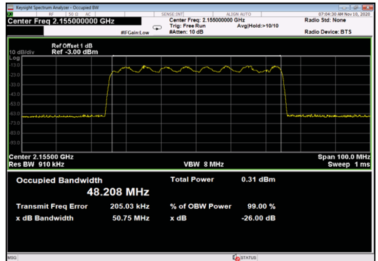
Figure 330: 16QAM 50MHz B.W.; 2155.0MHz, 15kHz - Input
