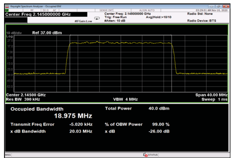
Figure 366: 64QAM 20MHz B.W.; 2145.0MHz, 15kHz - Input
