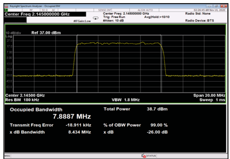
Figure 350: 64QAM 10MHz B.W.; 2145.0MHz, 60kHz - Input
