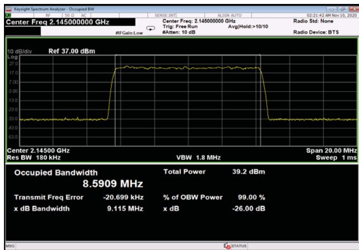
Figure 349: 64QAM 10MHz B.W.; 2145.0MHz, 30kHz - Input
