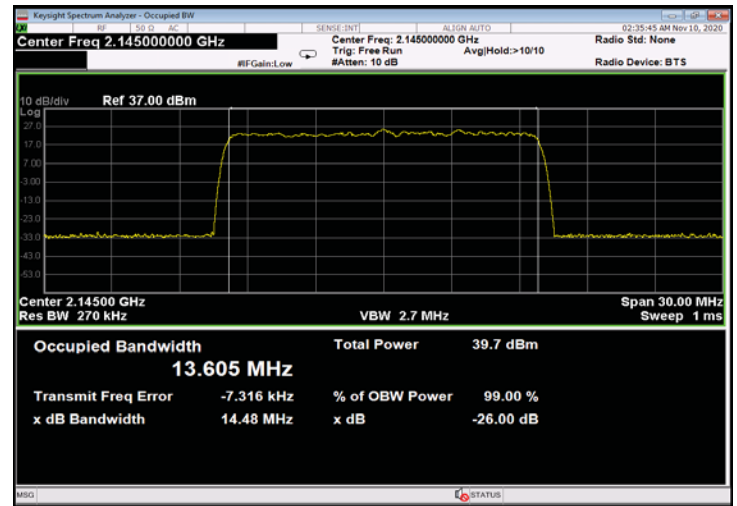
Figure 358: 64QAM 15MHz B.W.; 2145.0MHz, 30kHz - Input
