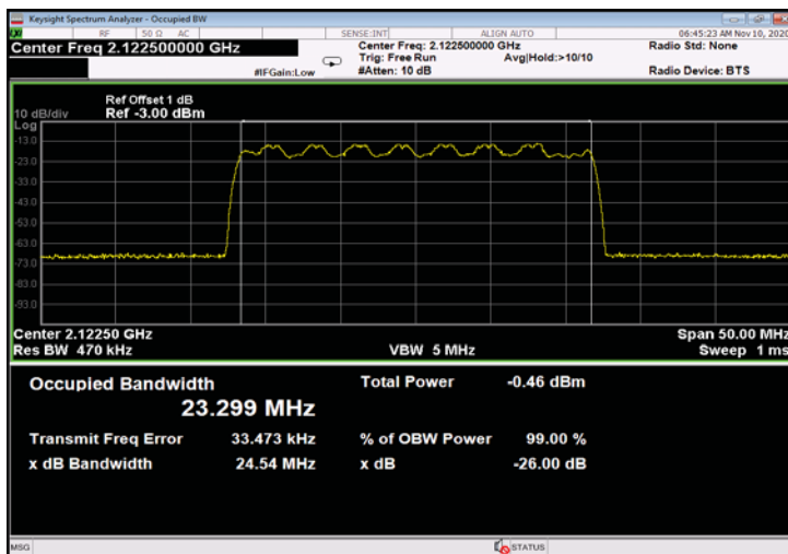
Figure 307: 16QAM 25MHz B.W.; 2122.5MHz, 30kHz - Input
