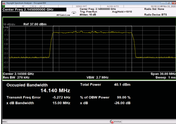
Figure 357: 64QAM 15MHz B.W.; 2145.0MHz, 15kHz - Input
