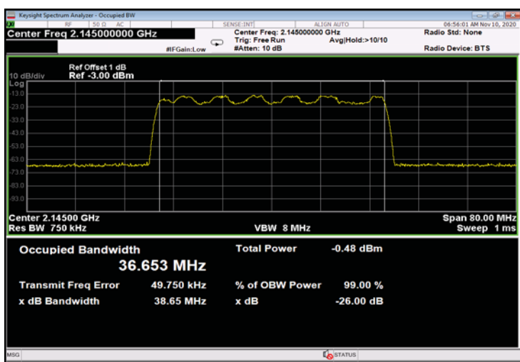
Figure 320: 16QAM 40MHz B.W.; 2145.0MHz, 60kHz - Input
