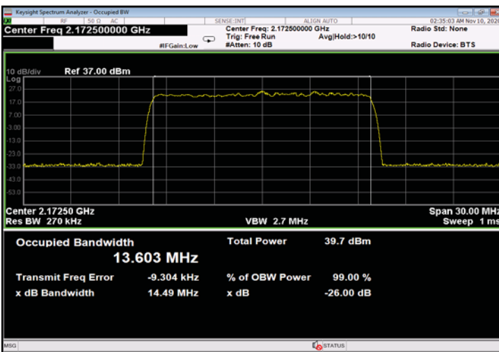
Figure 361: 64QAM 15MHz B.W.; 2172.5MHz, 30kHz - Input
