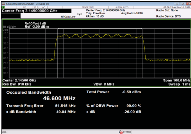
Figure 329: 16QAM 50MHz B.W.; 2145.0MHz, 60kHz - Input
