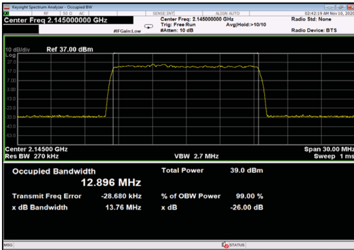
Figure 359: 64QAM 15MHz B.W.; 2145.0MHz, 60kHz - Input
