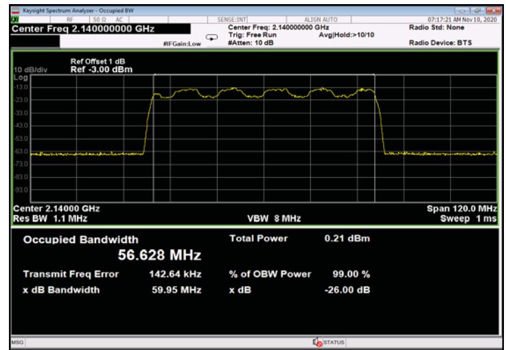
Figure 334: 16QAM 60MHz B.W.; 2140.0MHz, 60kHz - Input
