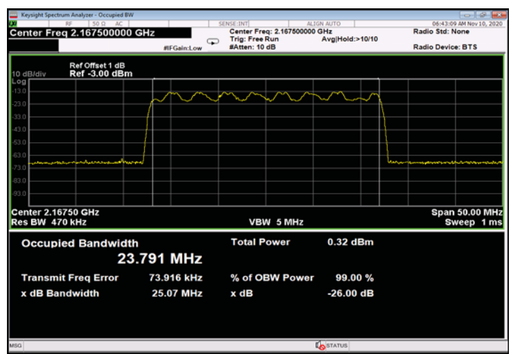
Figure 312: 16QAM 25MHz B.W.; 2167.5MHz, 15kHz - Input
