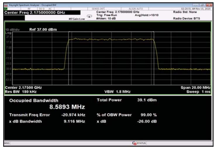
Figure 352: 64QAM 10MHz B.W.; 2175.0MHz, 30kHz - Input
