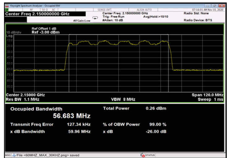
Figure 338: 16QAM 60MHz B.W.; 2150.0MHz, 60kHz - Input
