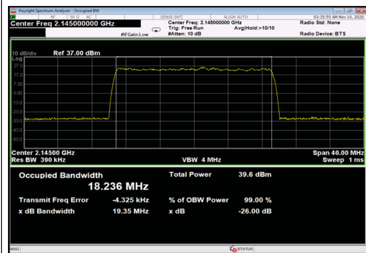
Figure 367: 64QAM 20MHz B.W.; 2145.0MHz, 30kHz - Input
