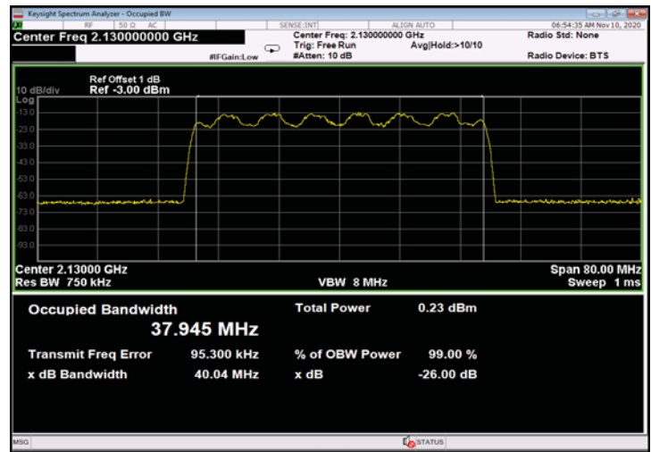
Figure 316: 16QAM 40MHz B.W.; 2130.0MHz, 30kHz - Input
