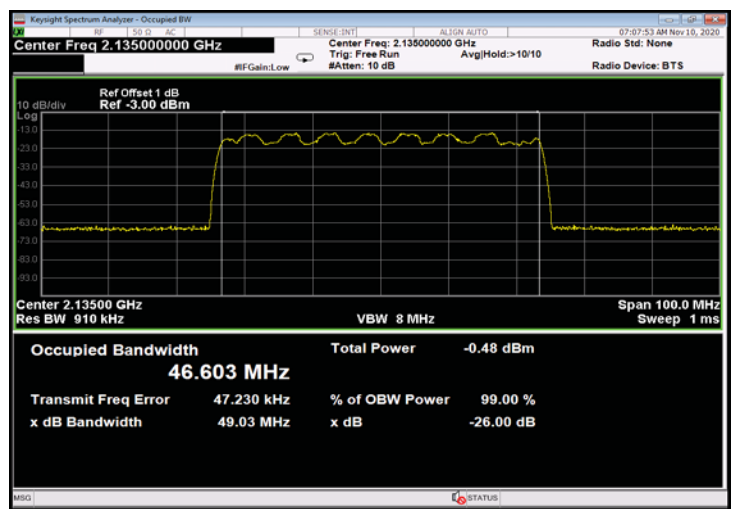
Figure 326: 16QAM 50MHz B.W.; 2135.0MHz, 60kHz - Input
