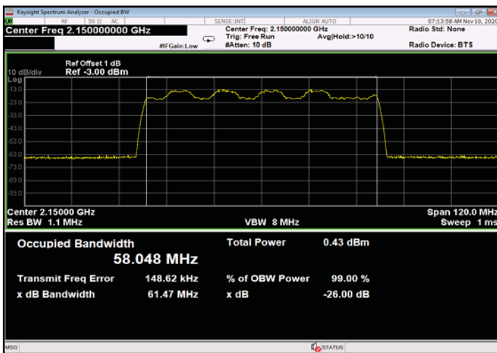
Figure 337: 16QAM 60MHz B.W.; 2150.0MHz, 30kHz - Input
