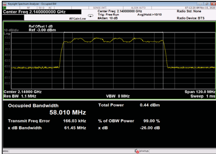
Figure 333: 16QAM 60MHz B.W.; 2140.0MHz, 30kHz - Input
