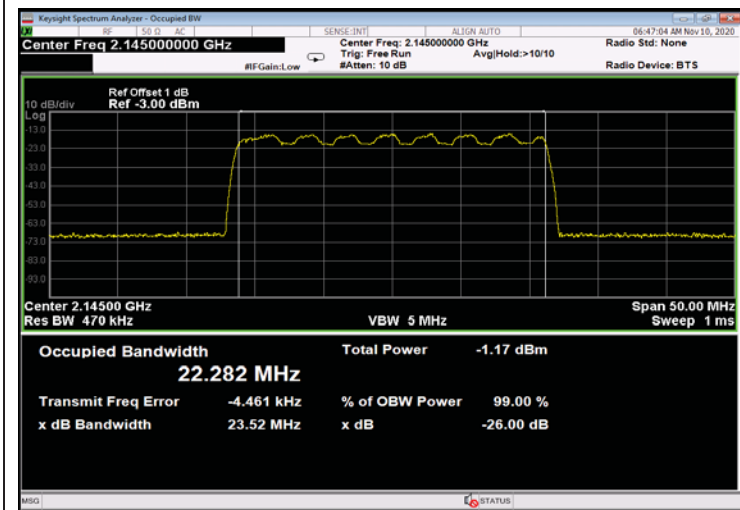
Figure 311: 16QAM 25MHz B.W.; 2145.0MHz, 60kHz - Input
