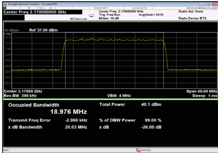
Figure 369: 64QAM 20MHz B.W.; 2170.0MHz, 15kHz - Input
