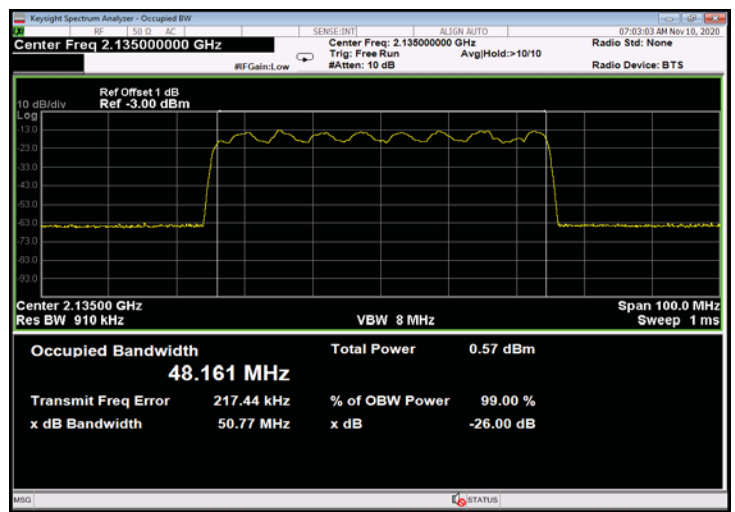
Figure 324: 16QAM 50MHz B.W.; 2135.0MHz, 15kHz - Input
