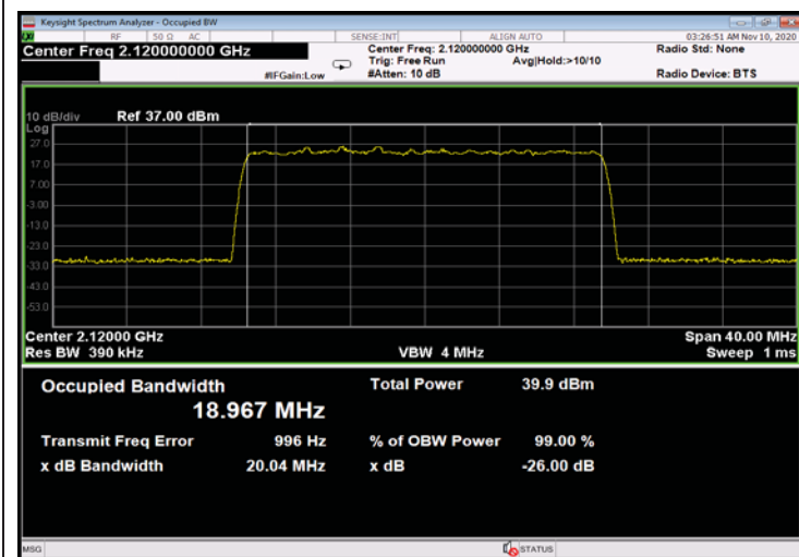
Figure 363: 64QAM 20MHz B.W.; 2120.0MHz, 15kHz - Input
