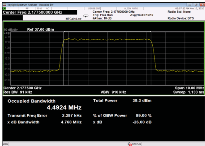
Figure 343: 64QAM 5MHz B.W.; 2177.5MHz, 15kHz - Input
