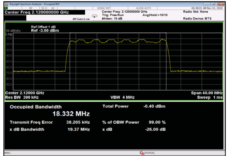
Figure 298: 16QAM 20MHz B.W.; 2120.0MHz, 30kHz - Input
