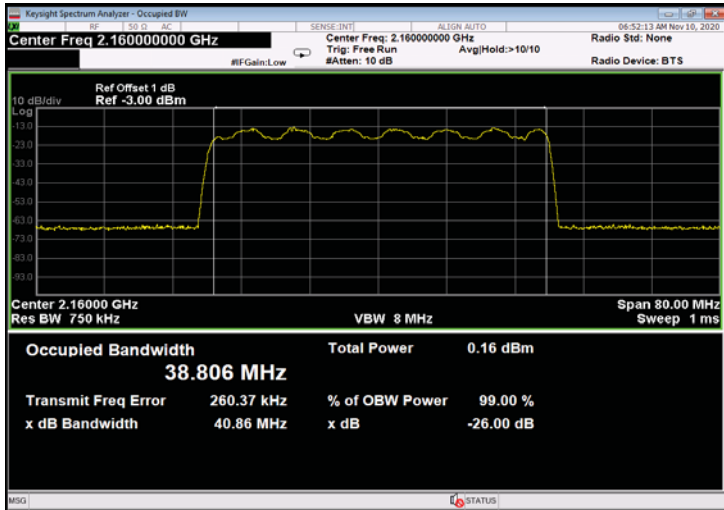
Figure 321: 16QAM 40MHz B.W.; 2160.0MHz, 15kHz - Input
