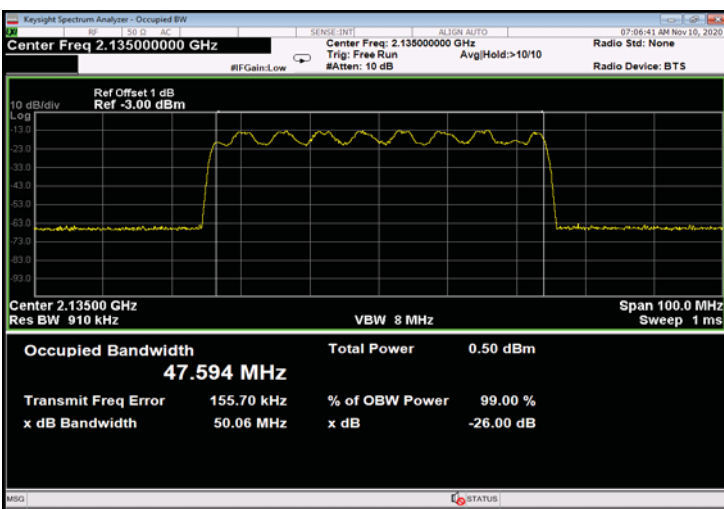
Figure 325: 16QAM 50MHz B.W.; 2135.0MHz, 30kHz - Input
