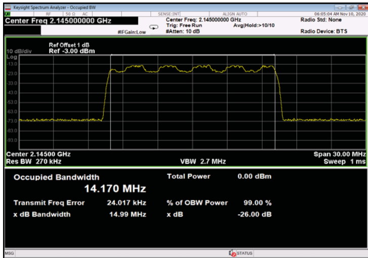
Figure 291: 16QAM 15MHz B.W.; 2145.0MHz, 15kHz - Input
