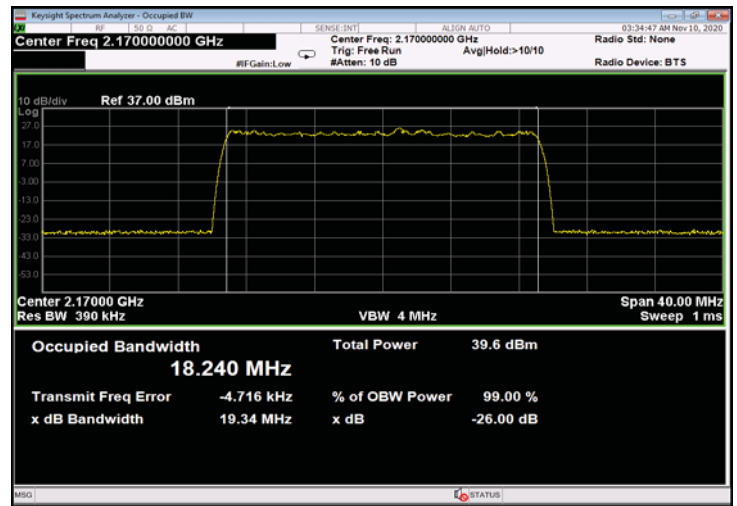
Figure 370: 64QAM 20MHz B.W.; 2170.0MHz, 30kHz - Input
