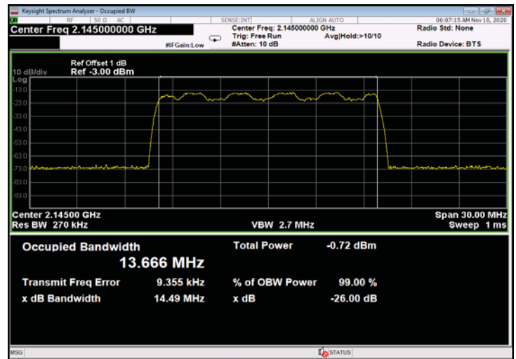
Figure 292: 16QAM 15MHz B.W.; 2145.0MHz, 30kHz - Input
