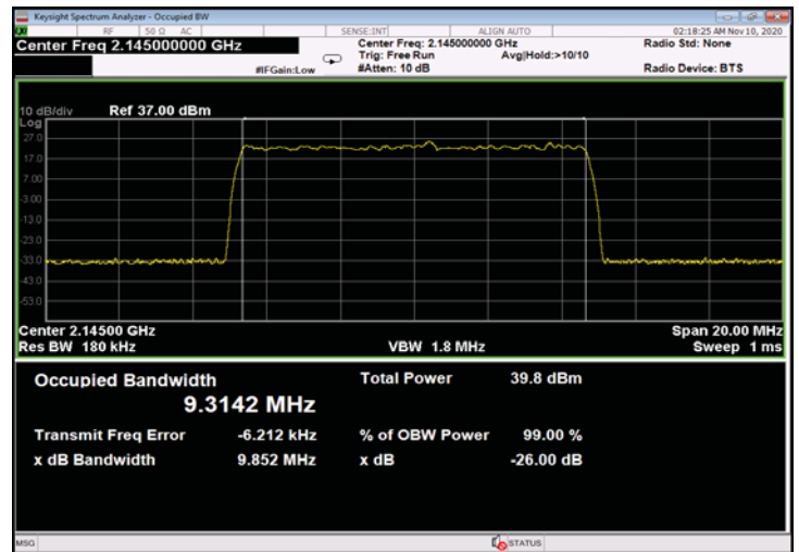
Figure 348: 64QAM 10MHz B.W.; 2145.0MHz, 15kHz - Input
