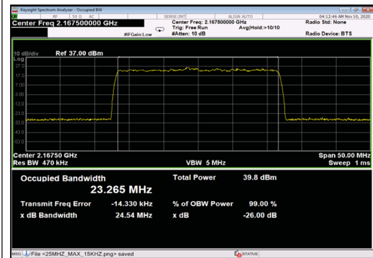
Figure 379: 64QAM 25MHz B.W.; 2167.5MHz, 30kHz - Input
