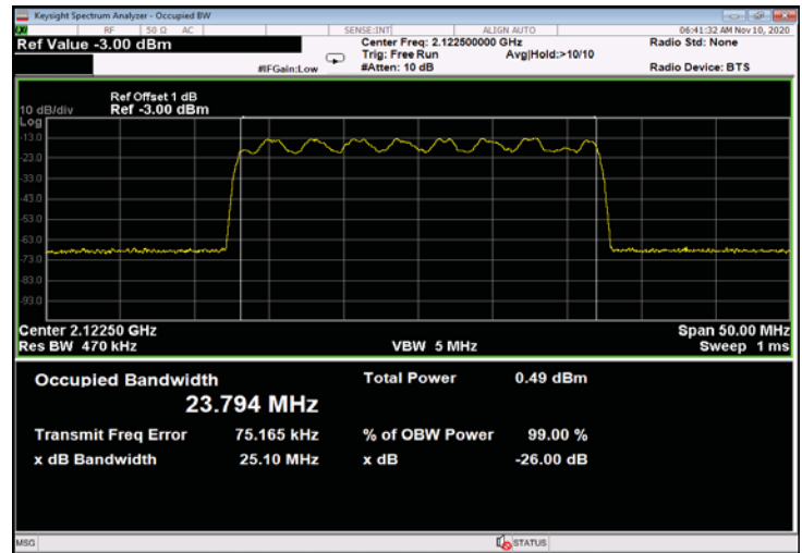
Figure 306: 16QAM 25MHz B.W.; 2122.5MHz, 15kHz - Input
