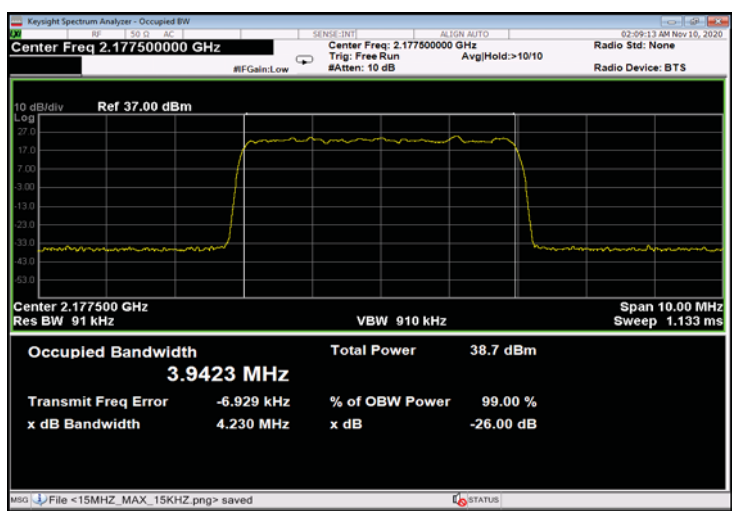
Figure 344: 64QAM 5MHz C.S.; 2177.5MHz, 30kHz - Input
