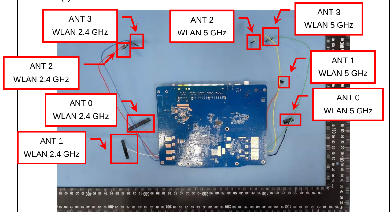
EUT Photo (4)
