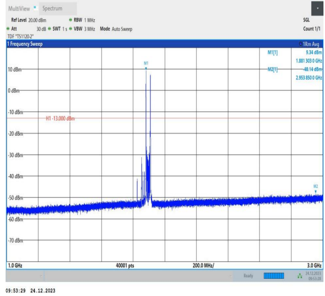
2-2-20MHz-10MHz-QPSK-QPSK-19001-19145-1RB#0-1RB#4 9-1000~3000MHz-PASS
