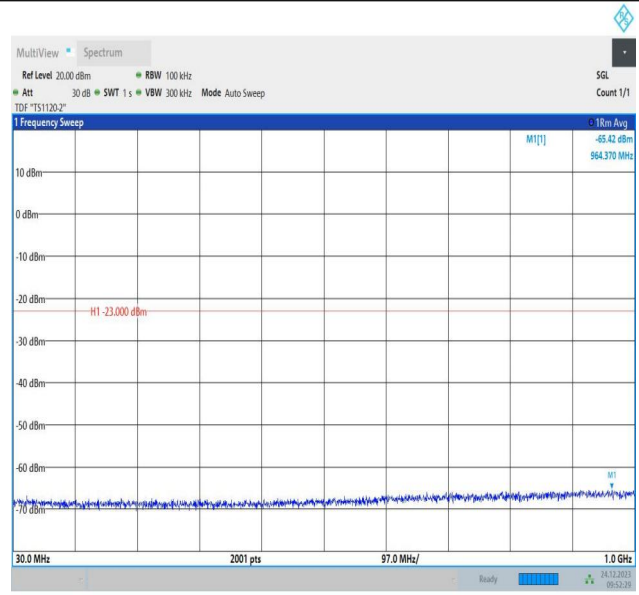
2-2-20MHz-10MHz-QPSK-QPSK-19001-19145-1RB#99-0RB# 0-30~1000MHz-PASS
