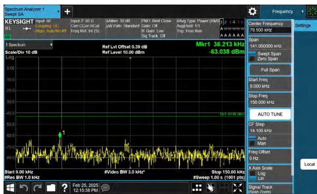
Band4-20MHz-QPSK-20175-1RB#0-0.009~0.15-PASS
