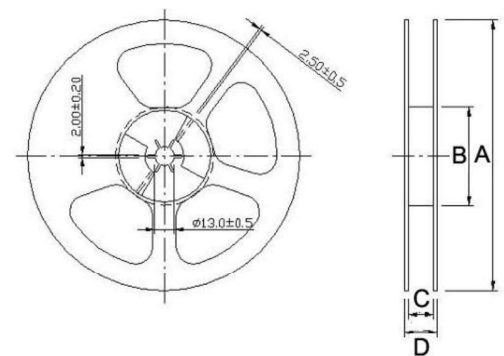
Reel Dimensions
