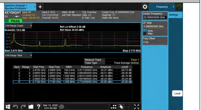
Band41-20MHz-QPSK-41490-1RB#0-PASS
