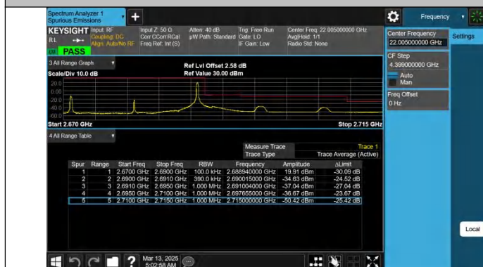
Band41-20MHz-QPSK-41490-1RB#99-PASS
