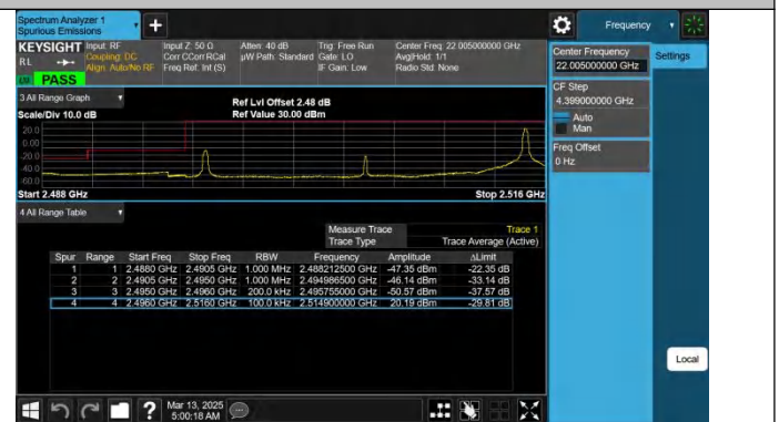
Band41-20MHz-QPSK-39750-1RB#99-PASS
