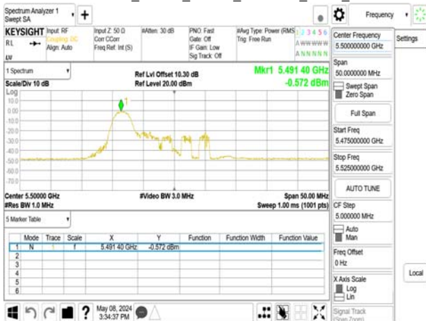
802.11be_20MHz_Chain1_5500MHz_RU26_0
