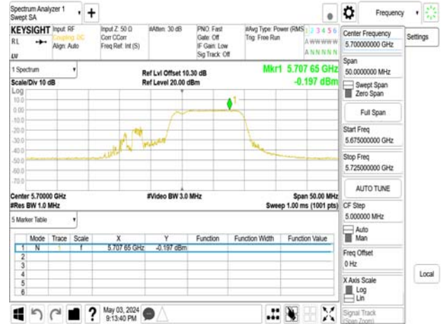
802.11be_20MHz_Chain0_5700MHz_52+26_MRU3
