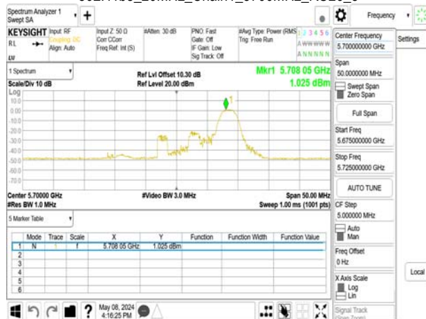
802.11be_20MHz_Chain1_5700MHz_RU52_40
