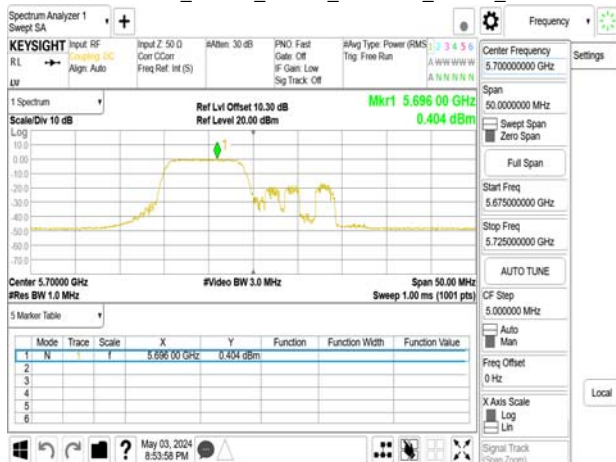
802.11be_20MHz_Chain1_5700MHz_RU106_54
