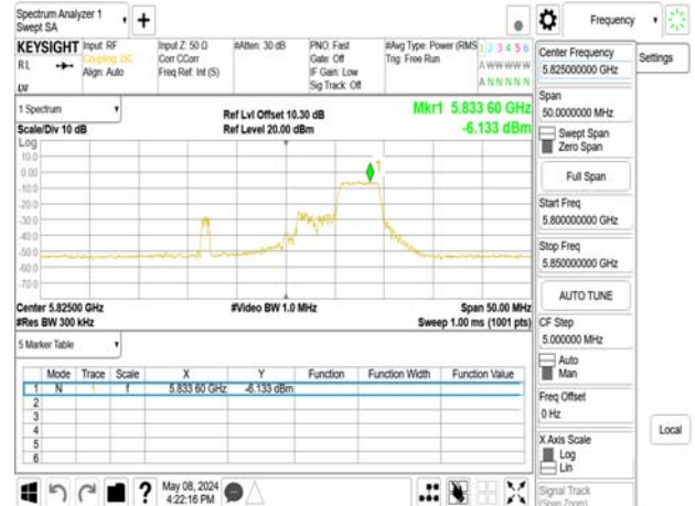
802.11be_20MHz_Chain0_5825MHz_RU52_40
