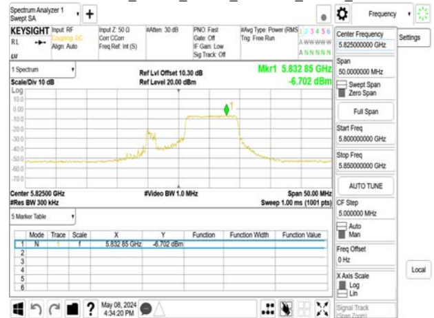
802.11be_20MHz_Chain0_5825MHz_RU26_8
