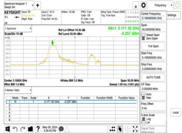
802.11be_20MHz_Chain1_5180MHz_RU52_37
