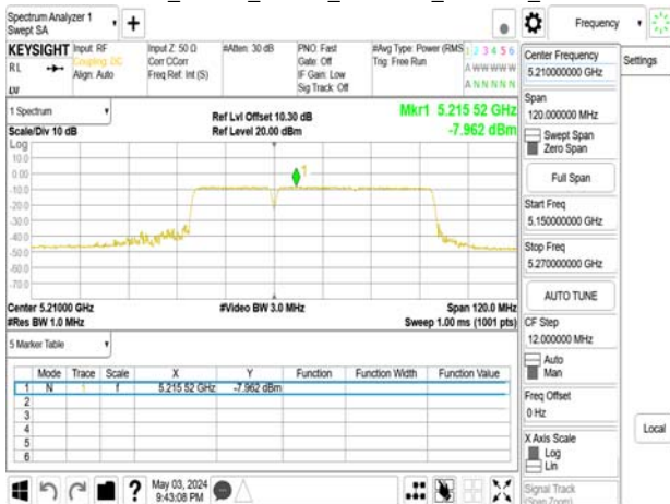
802.11be_80MHz_Chain1_5210MHz_484+242_MRU1
