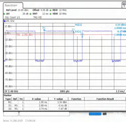
NTNV-2DH5-Ant1-2480
