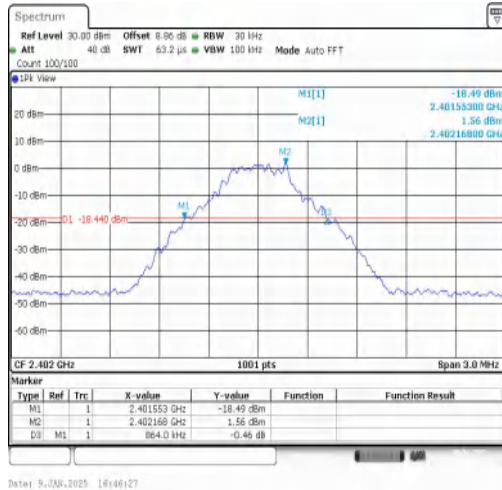
DH5-Ant1-2402
