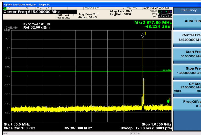
Band5-5MHz-QPSK-20425-1RB#0-30~1000MHz
