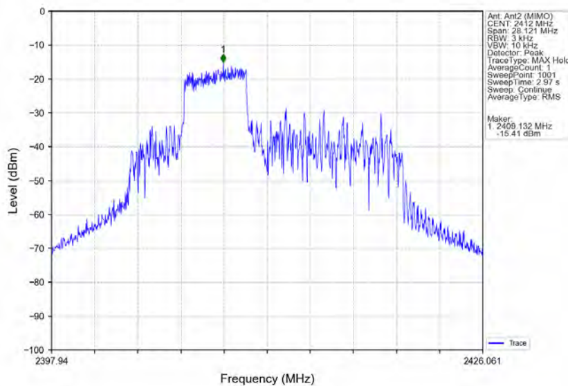
802.11ax(HE20) LCH 2412MHz RU52 Mid Ant2 (MIMO) NTN
