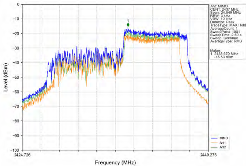
802.11ax(HE20) MCH 2437MHz RU242 Left Ant1 (MIMO) NTN
