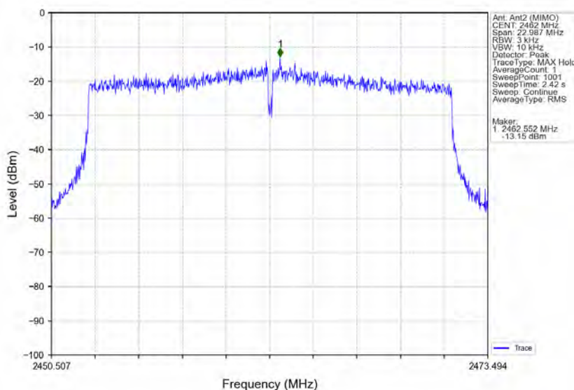
802.11ax(HE20) HCH 2462MHz RU242 Left Ant2 (MIMO) NTNV
