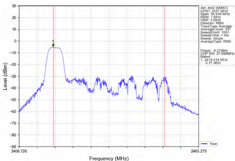
802.11ax(HE40) MCH 2437MHz RU52 Left Ant2 (MIMO) NTVN
