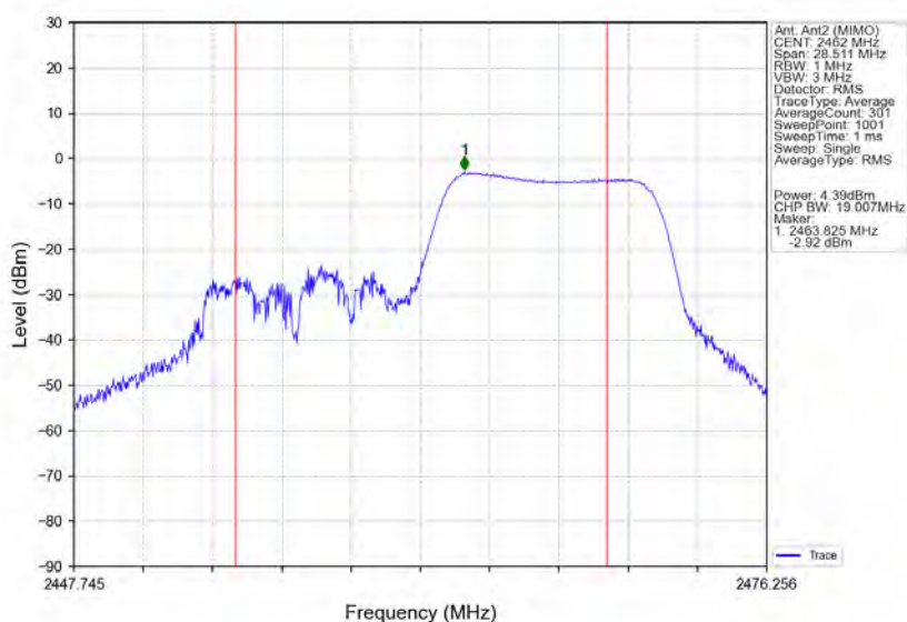
802.11ax(HE20) HCH 2462MHz RU106 Right Ant2 (MIMO) NTNW
