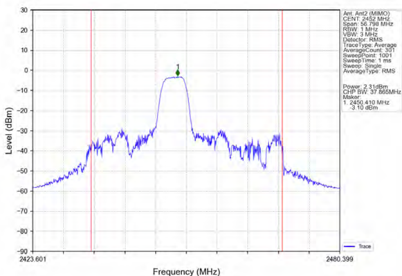
802.11ax(HE40) HCH 2452MHz RU52 Mid Ant2 (MIMO) NTVN
