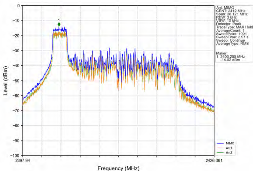
802.11ax(HE20) LCH 2412MHz RU26 Mid Ant1 (MIMO) NTN
