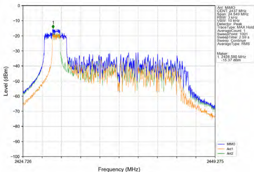
802.11ax(HE20) MCH 2437MHz RU26 Left MIMO NTNV
