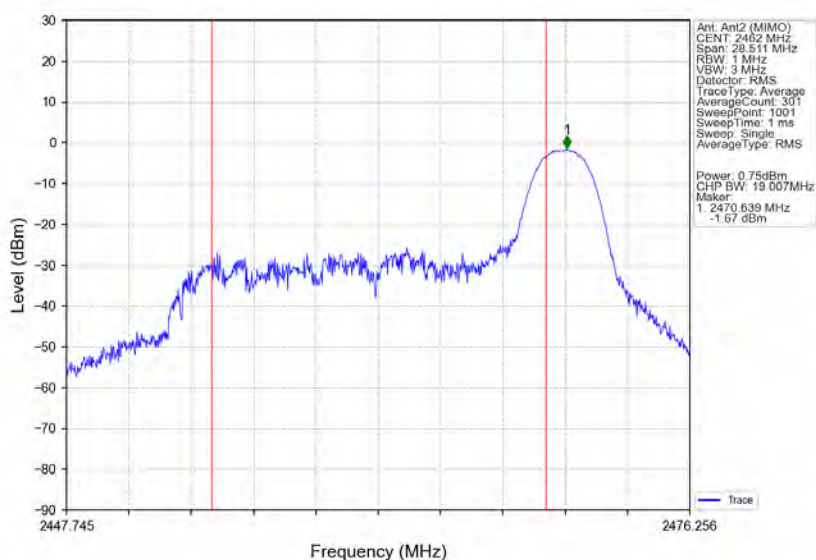
802.11ax(HE20) HCH 2462MHz RU26 Right Ant2 (MIMO) NTNv
