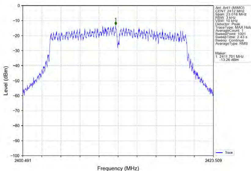
802.11g LCH 2412MHz Ant1 (MIMO) NTN
