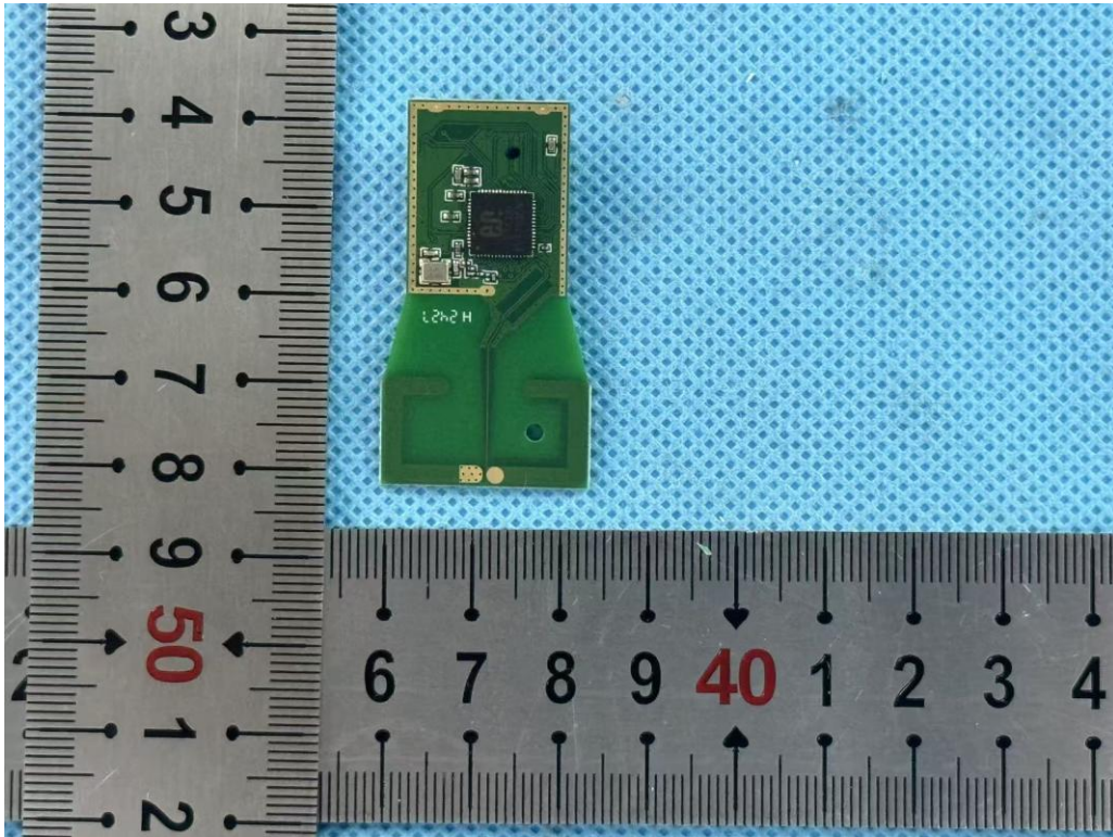
2.4G ANT
