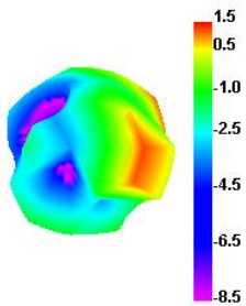
5150.000MHz E1
