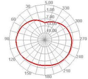
2400.000MHz H
