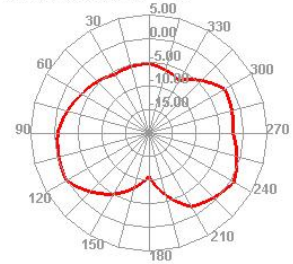
2400.000MHz E2
