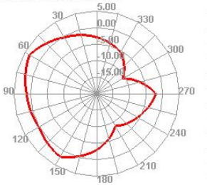
5800.000MHz E1
