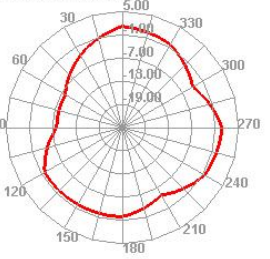
5800.000MHz H
