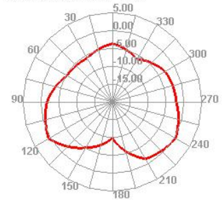
2500.000MHz E2
