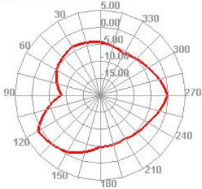
5450.000MHz E2
