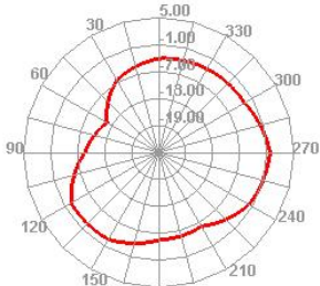
5450.000MHz H
