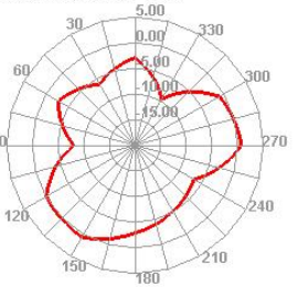
5800.000MHz E2
