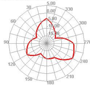
2500.000MHz E1
