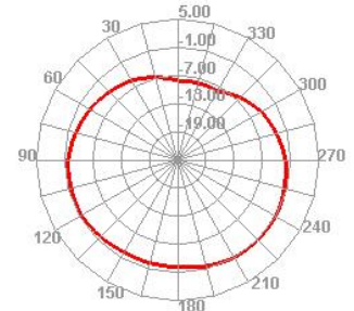
2500.000MHz H
