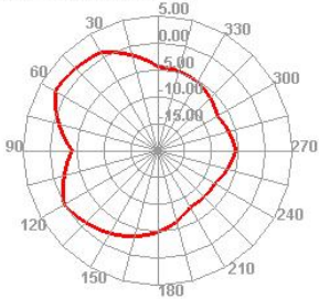
5450.000MHz E1
