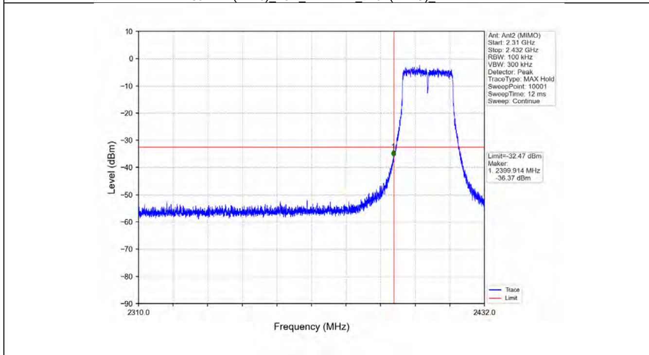
802.11n(HT20)_LCH_2412MHz_Ant2 (MIMO)_NTNV
