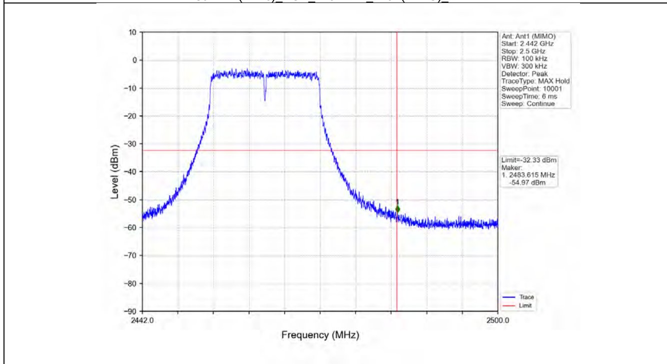
802.11n(HT20)_HCH_2462MHz_Ant1 (MIMO)_NTNV
