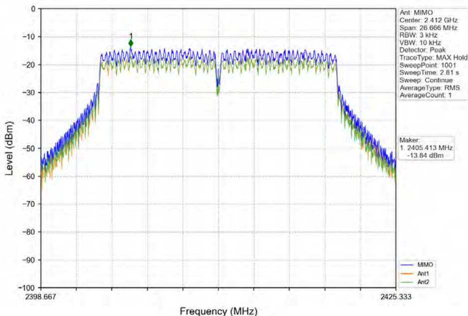
802.11n(HT20)_LCH_2412MHz_MIMO _NTNV
