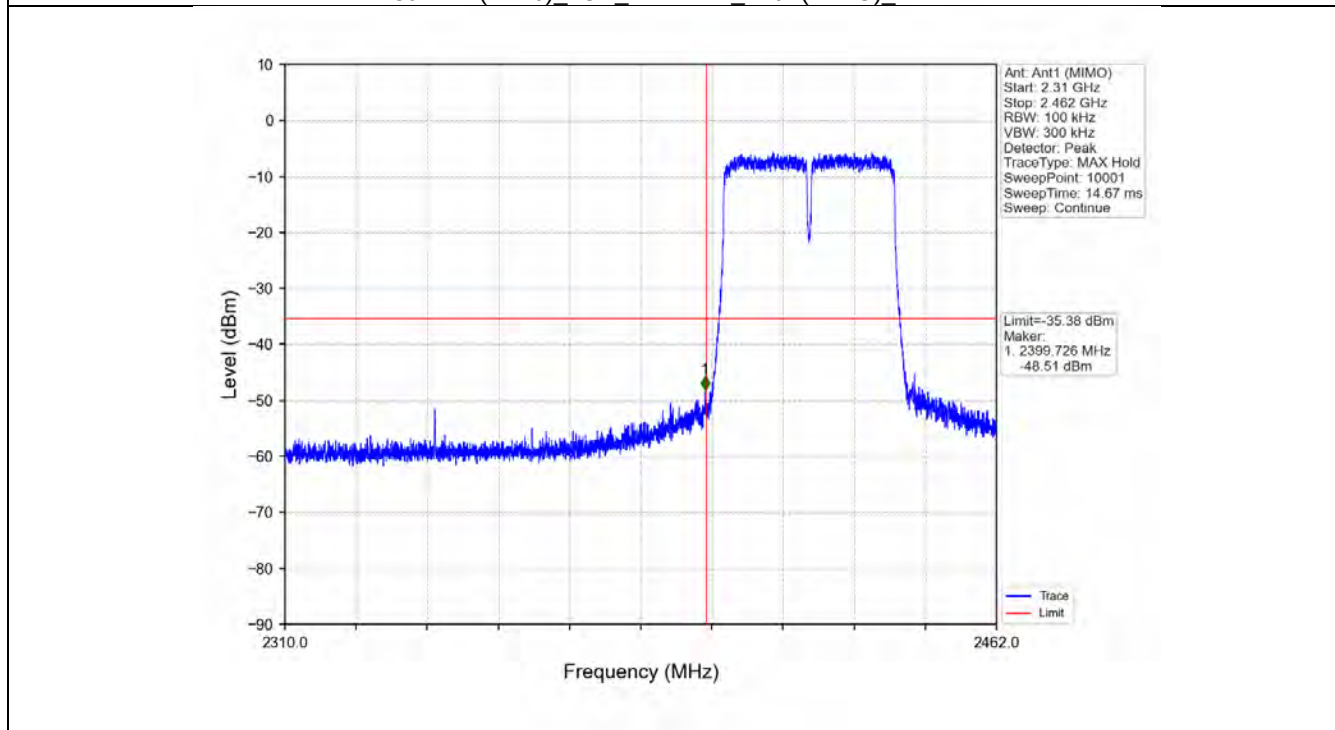
802.11n(HT40)_LCH_2422MHz_Ant1 (MIMO)_NTNV
