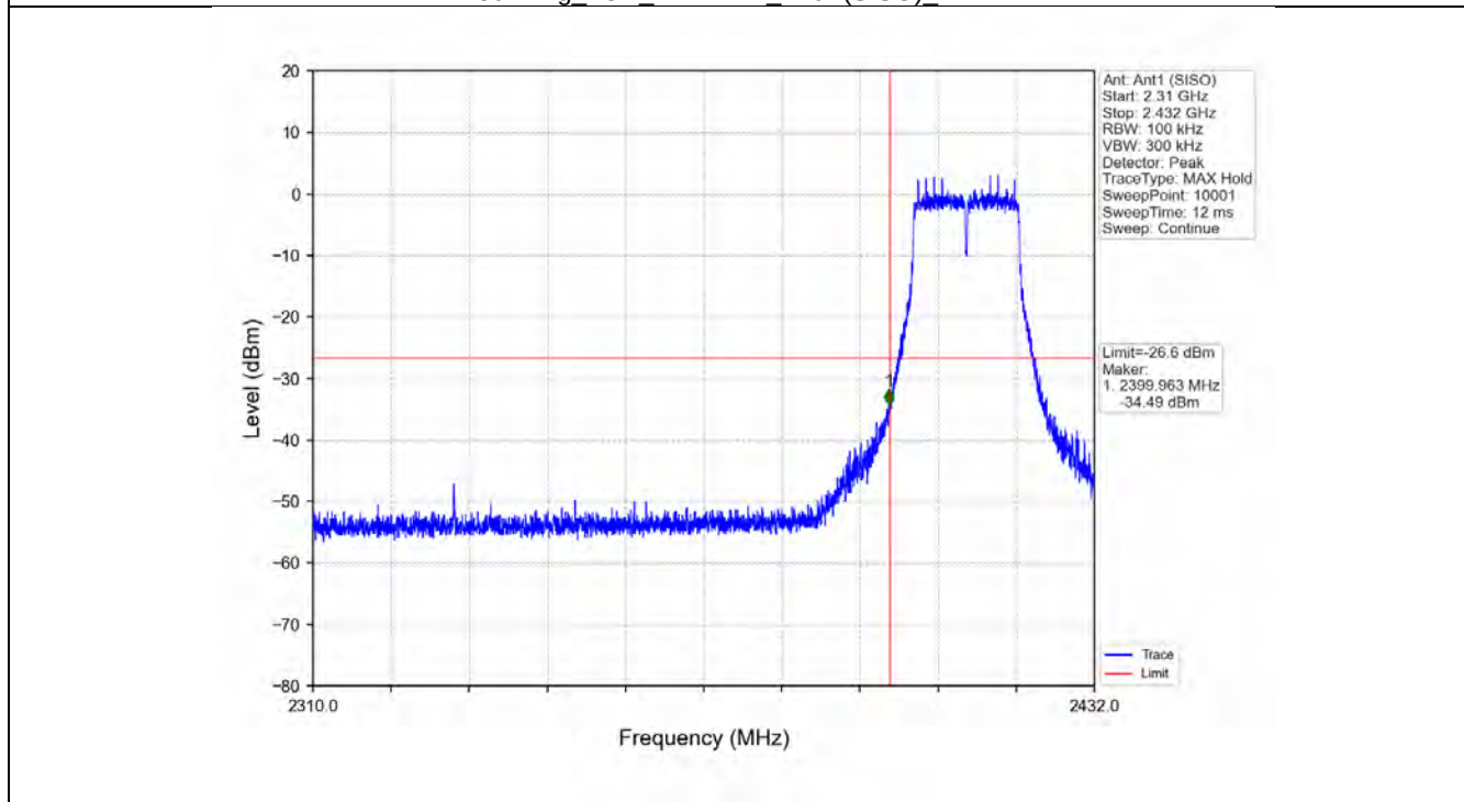
802.11g_LCH_2412MHz_Ant1 (SISO)_NTNV
