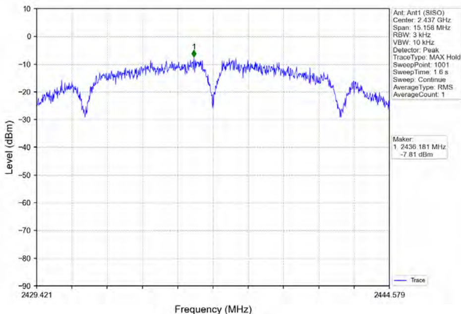
802.11b MCH 2437MHz Ant1 (SISO) NTV
