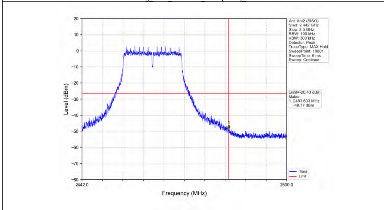
802.11g_HCH_2462MHz_Ant2 (SISO)_NTNV
