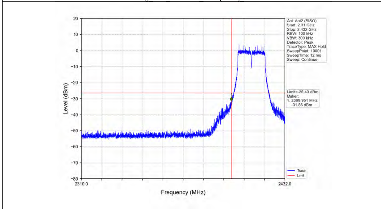
802.11g_LCH_2412MHz_Ant2 (SISO)_NTNV
