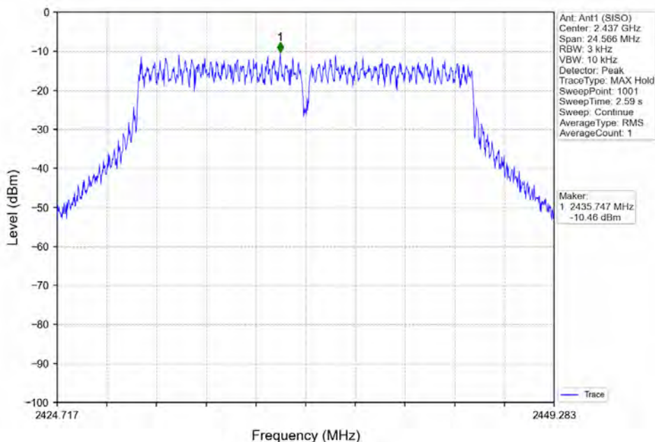
802.11g MCH 2437MHz Ant1 (SISO) NTVN
