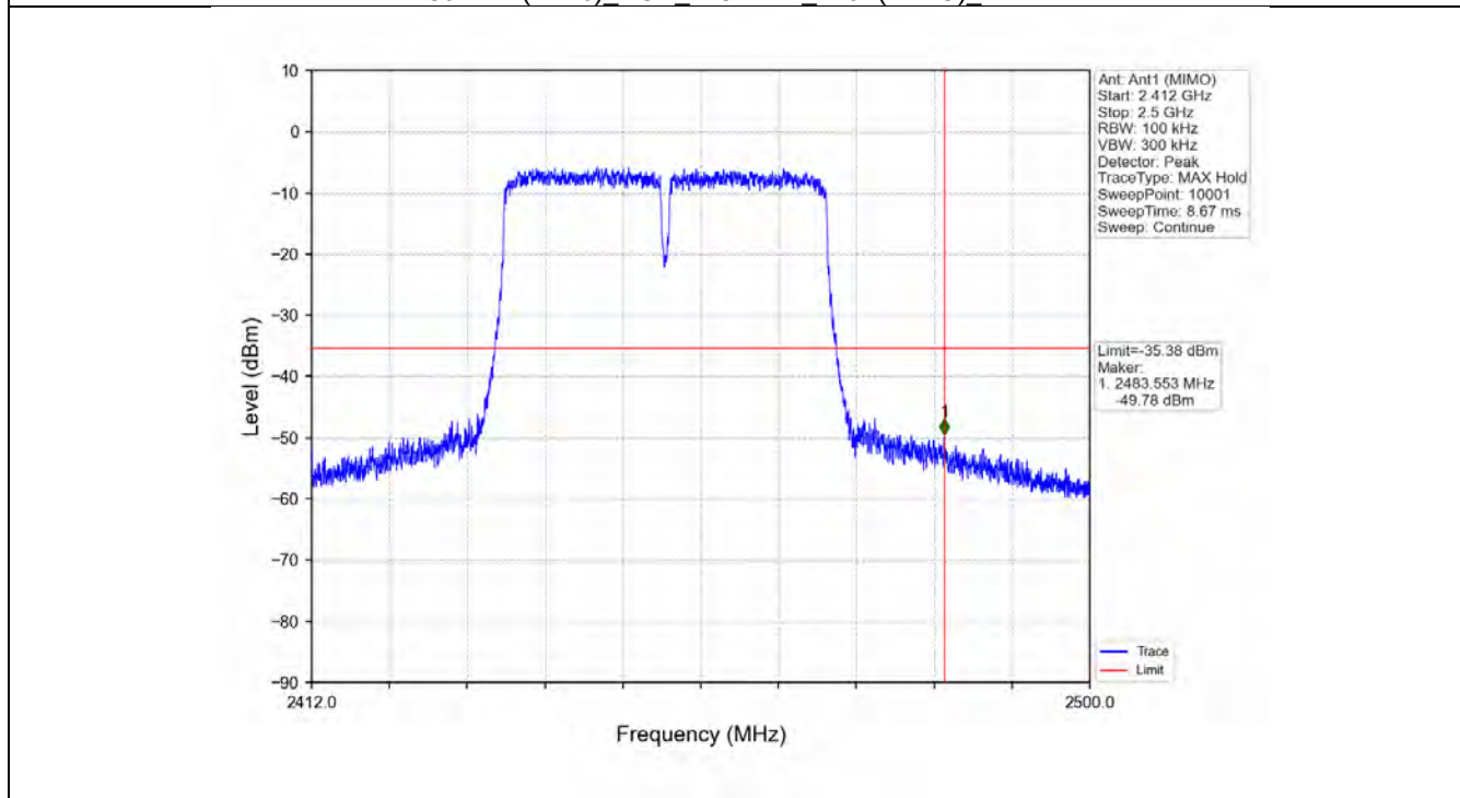
802.11n(HT40)_HCH_2452MHz_Ant1 (MIMO)_NTNV
