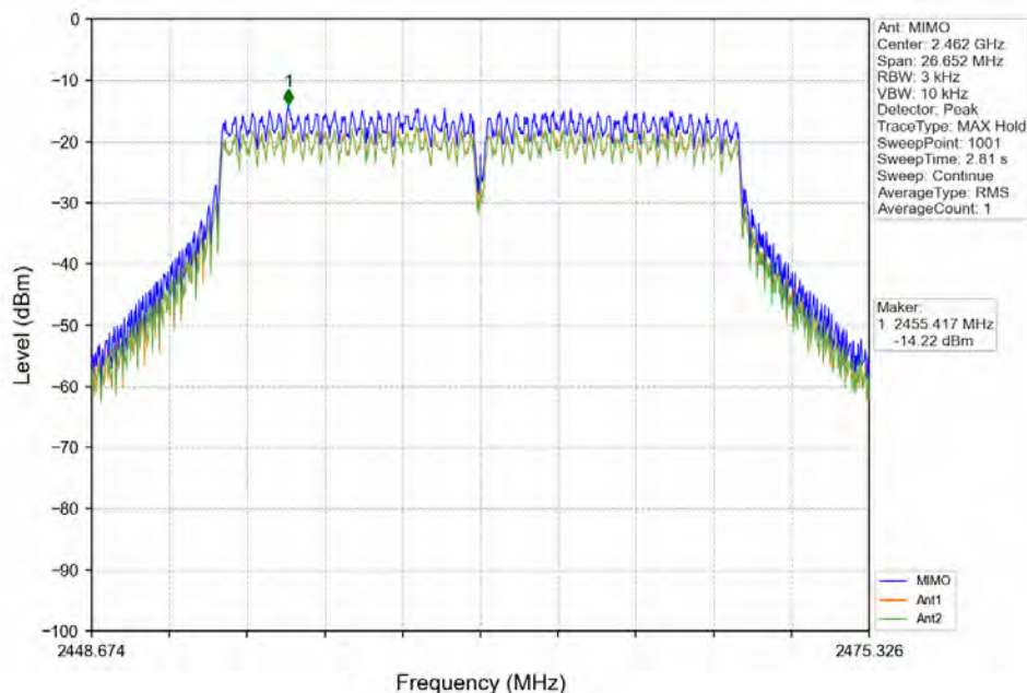
802.11n(HT20) HCH 2462MHz MIMO NTN
