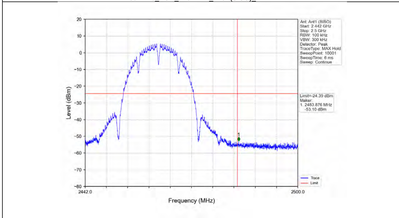
802.11b_HCH_2462MHz_Ant1 (SISO)_NTNV
