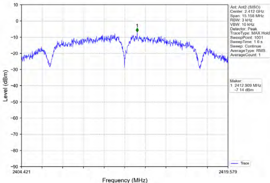
802.11b LCH 2412MHz Ant2 (SISO) NTV
