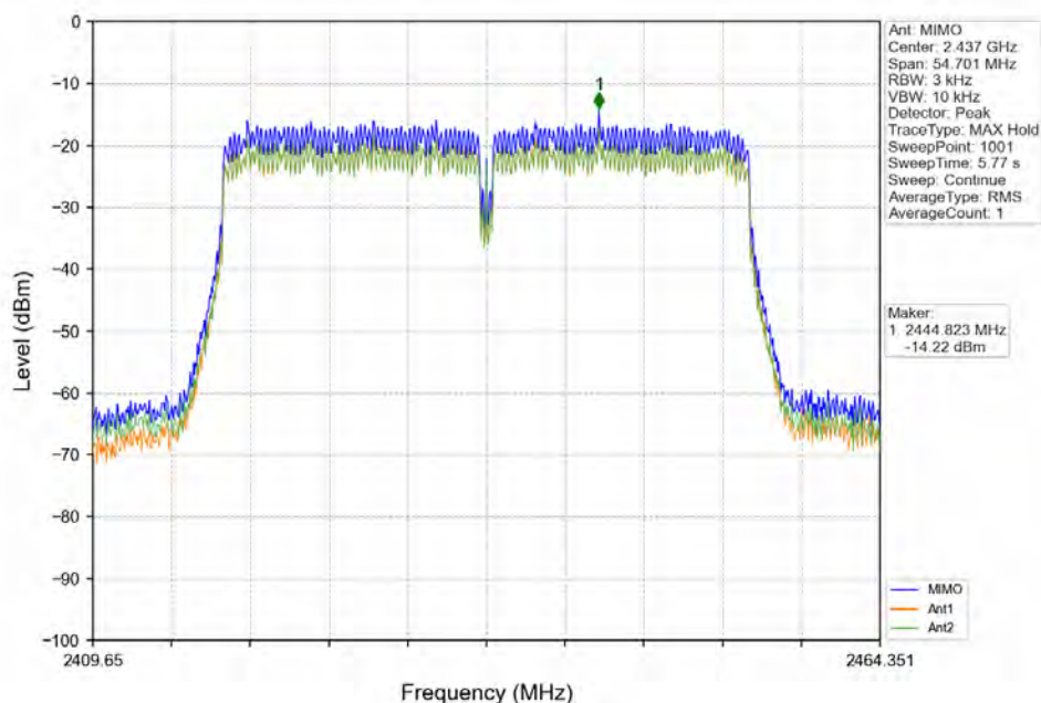
802.11n(HT40) MCH 2437MHz MIMO NTNV
