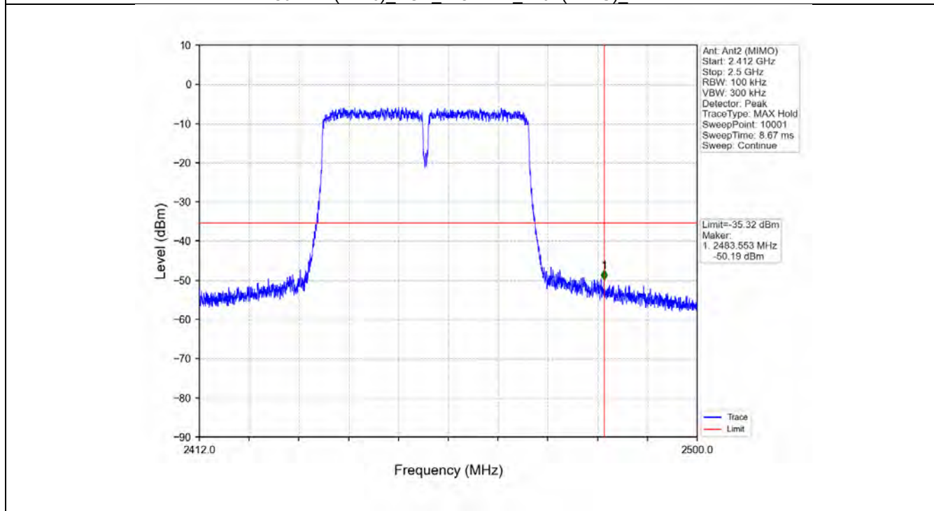
802.11n(HT40)_HCH_2452MHz_Ant2 (MIMO)_NTNV
