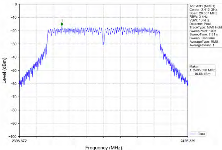
802.11n(HT20) LCH 2412MHz Ant1 (MIMO) NTN
