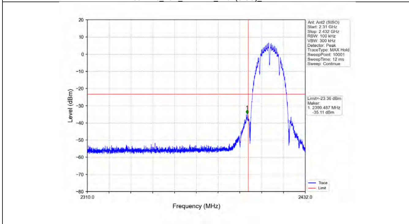
802.11b_LCH_2412MHz_Ant2 (SISO)_NTNV
