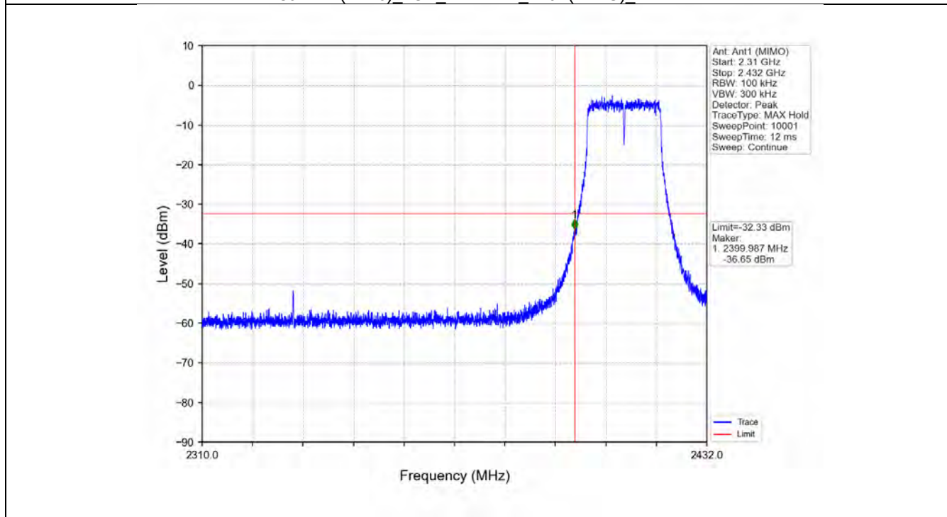
802.11n(HT20)_LCH_2412MHz_Ant1 (MIMO)_NTNV
