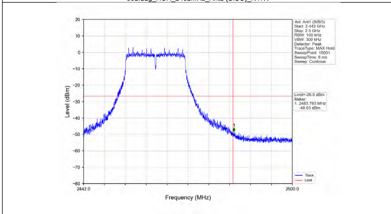
802.11g_HCH_2462MHz_Ant1 (SISO)_NTNV
