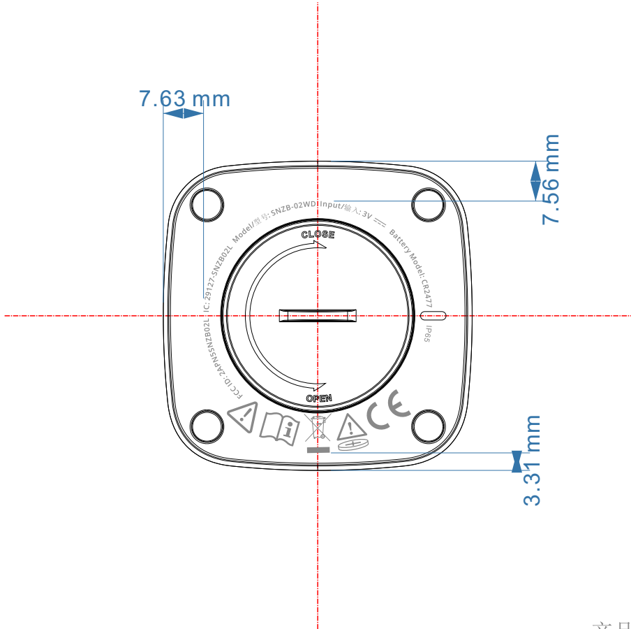
镭雕位置
