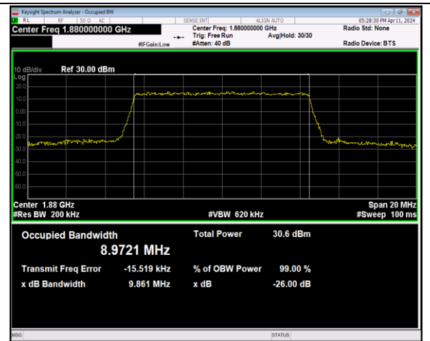
Band2-10MHz-16QAM-18900-50RB#0-PASS
