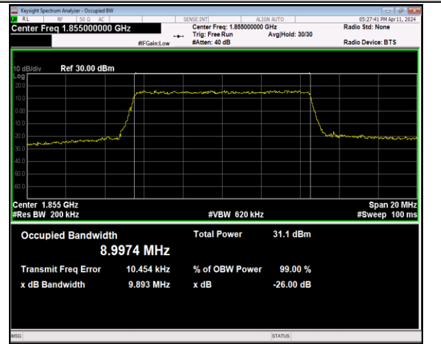
Band2-10MHz-QPSK-18650-50RB#0-PASS
