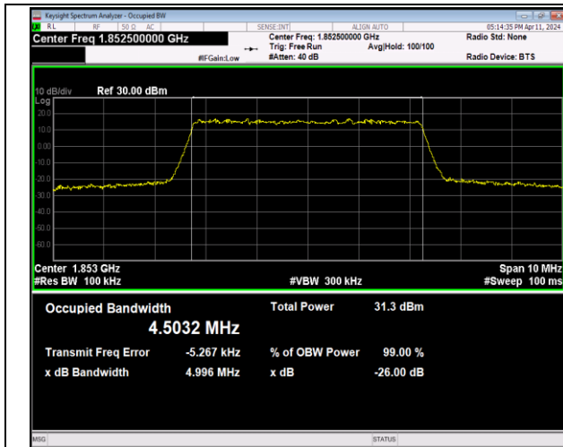
Band2-5MHz-QPSK-18625-25RB#0-PASS
