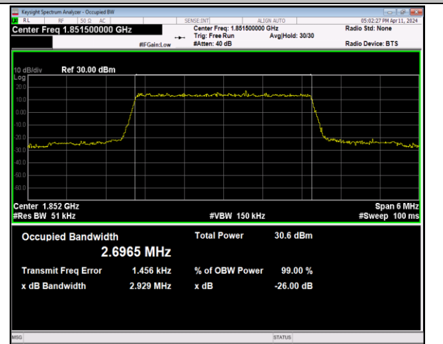
Band2-3MHz-QPSK-18615-15RB#0-PASS
