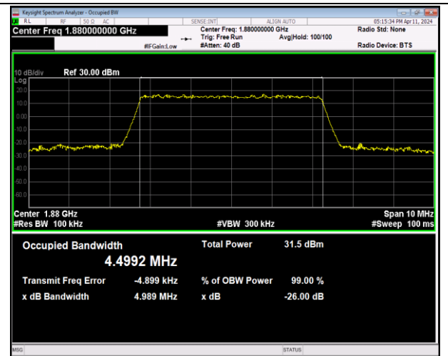
Band2-5MHz-QPSK-18900-25RB#0-PASS
