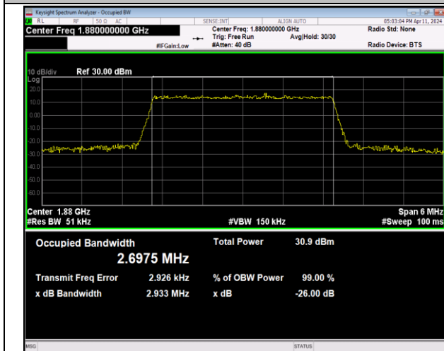
Band2-3MHz-QPSK-18900-15RB#0-PASS
