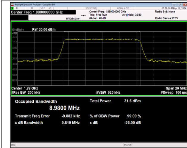
Band2-10MHz-QPSK-18900-50RB#0-PASS
