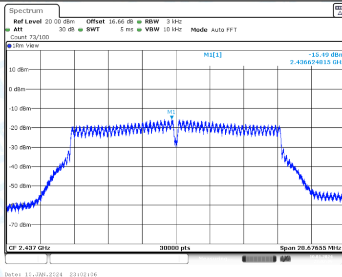
11N20-CDD_Ant2_2437
