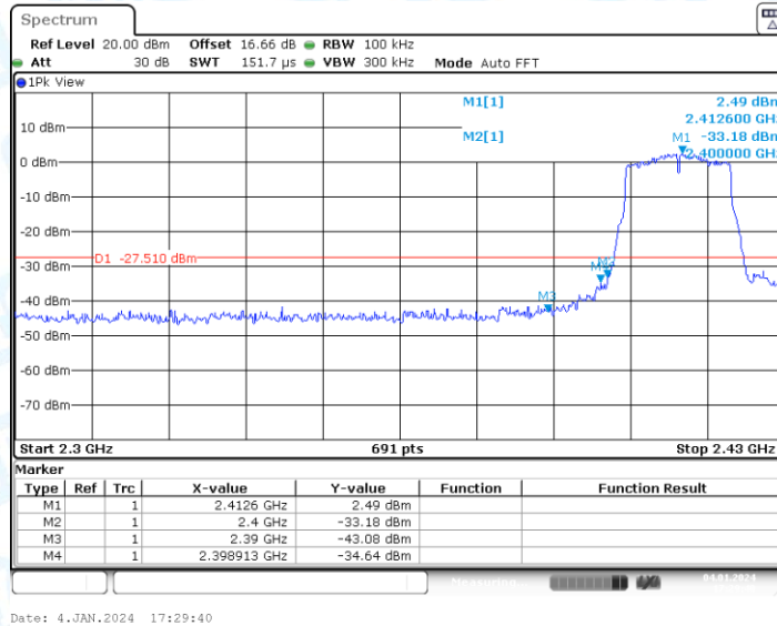
11N20-CDD_Ant2_Low_2412
