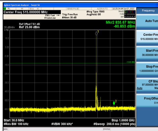
Band12-3MHz-QPSK-23025-1-0-Low-30-1000--60.85-PASS
