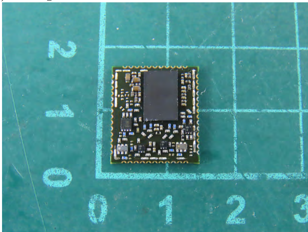
(14) EUT Photo_ RF Module
