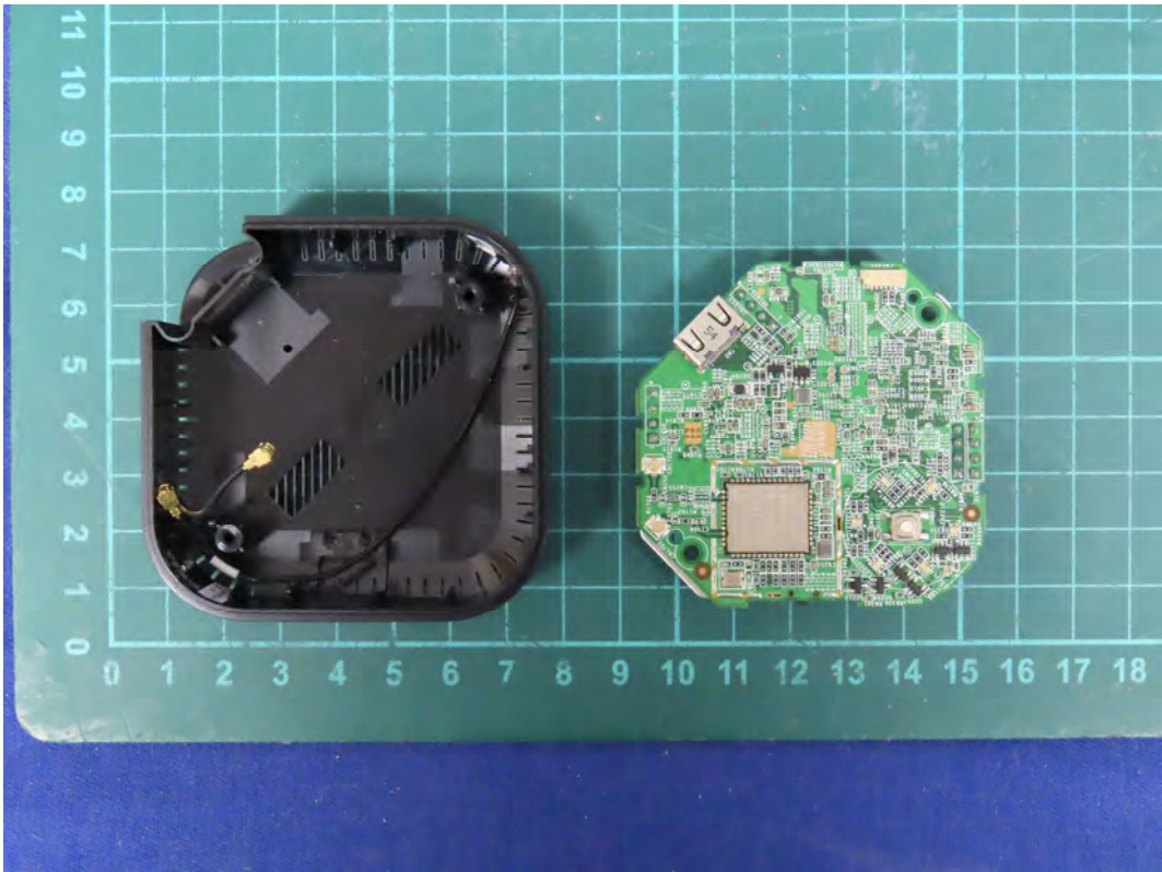
(9) EUT Photo
