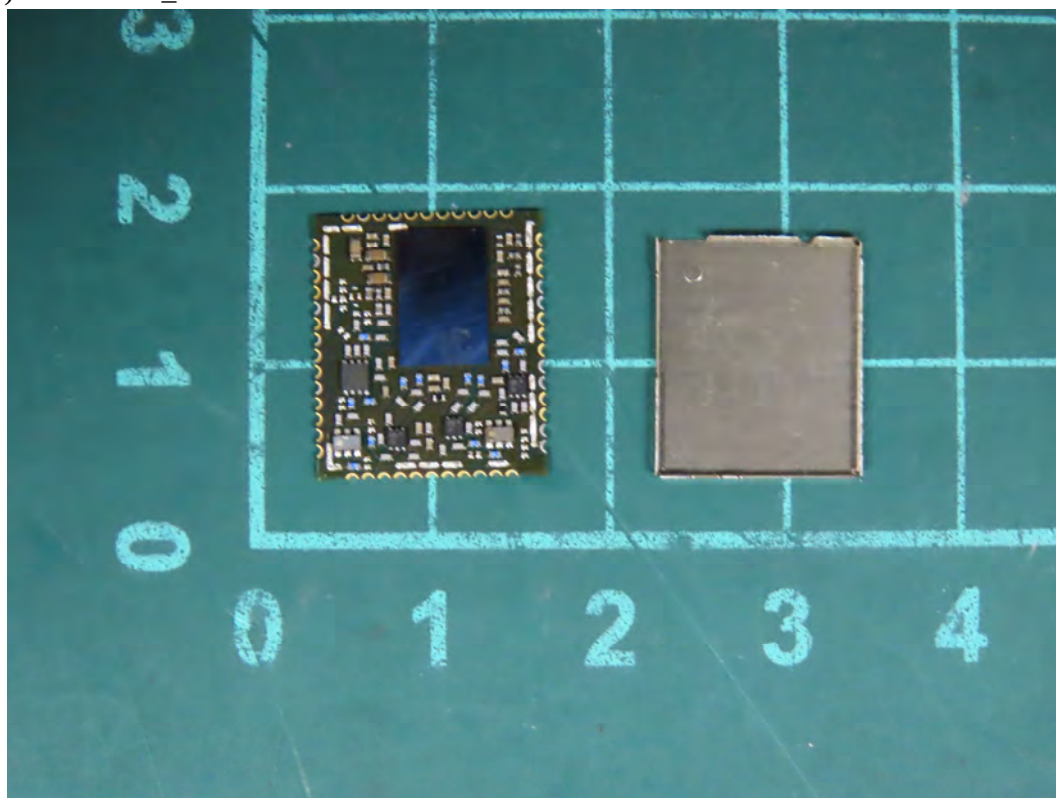
(13) EUT Photo_RF Module
