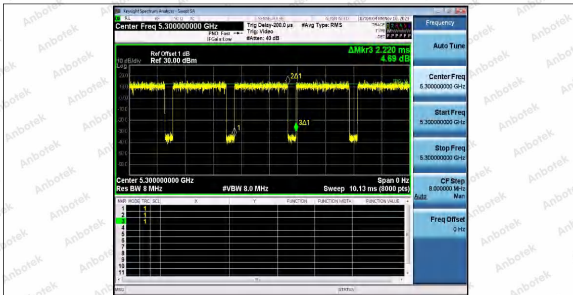
11N20SISO_Ant2_5300
