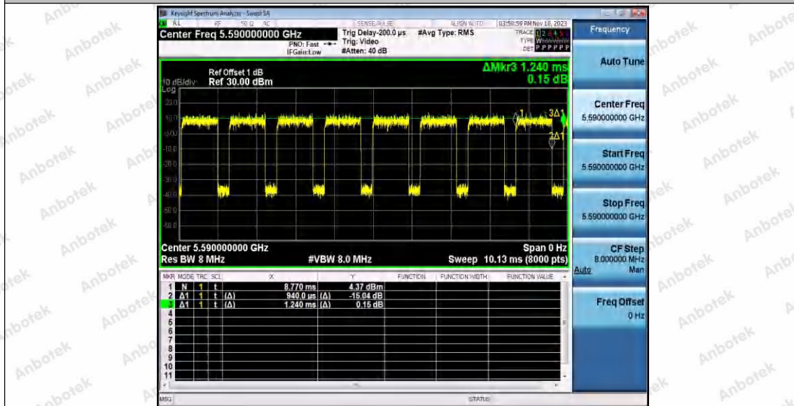
11N40SISO_Ant2_5590
