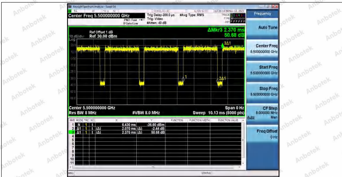
11A_Ant2_5500
