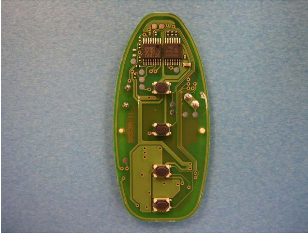
PCB Top
