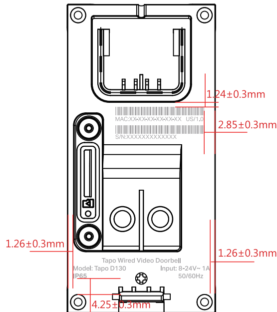
底壳尺寸图
