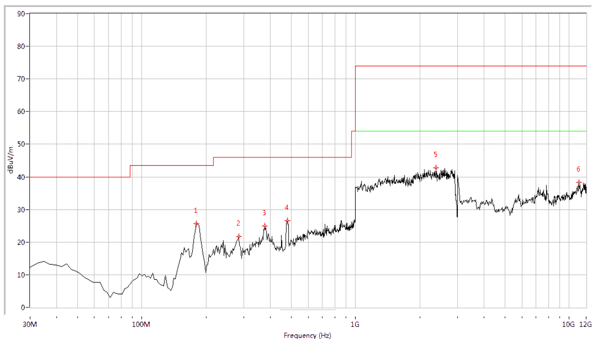
(Plot B: 30MHz – 12GHz, Test Antenna Horizontal)
