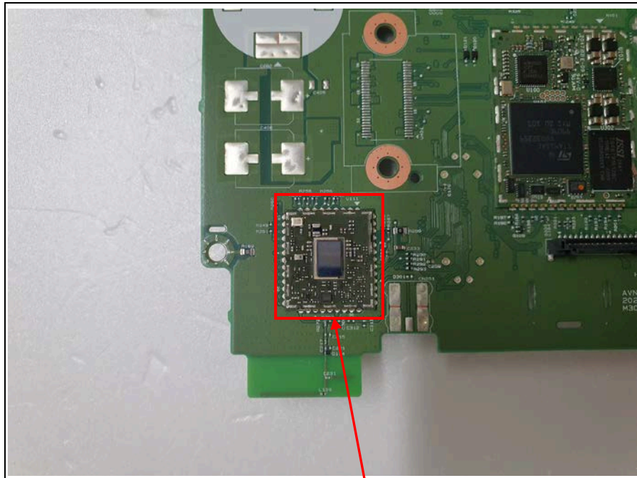
BT/WIFI Module
